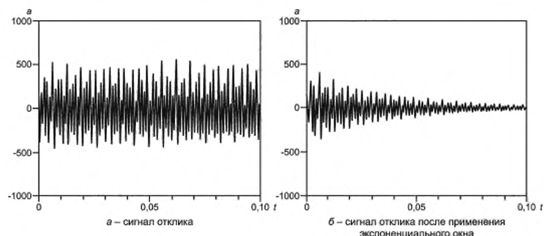
Рисунок 7 — Сигналы отклика без применения и с применением экспоненциального окна и полученные для них графики ускорения
