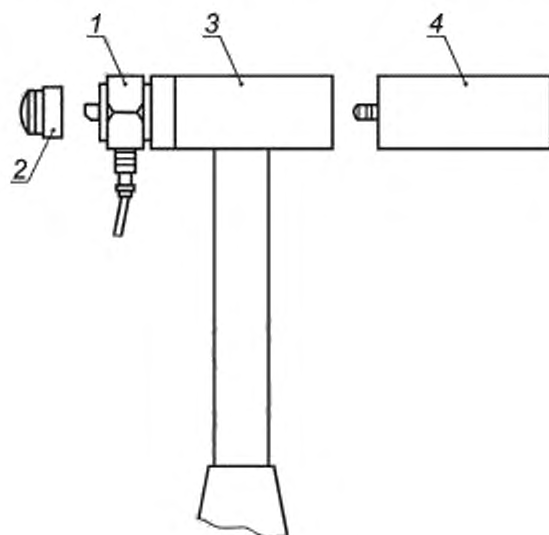
1 — преобразователь силы; 2 — сменная насадка; 3 — основная масса; 4 — сменная масса
