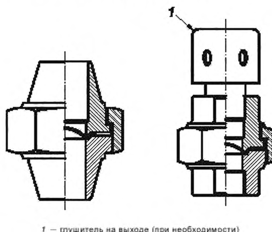
Рисунок 7 — Типовые держатели разрывных мембран в виде штуцера
