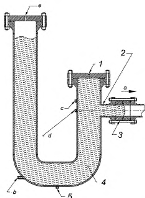
1 — отверстие для сброса воздуха после заполнения жидкостью; 2 — номинальный диаметр трубопровода должен быть больше или равен номинальному диаметру устройства с разрывной мембраной; 3 — устройство с разрывной мембраной; 4 — несжимаемая среда; 5 — дренажная пробка; а — поток испытательной среды; б — подвод среды; с — датчик температуры; d — место измерения давления на линии оси устройства с разрывной мембраной; е — подача газа (пара)
