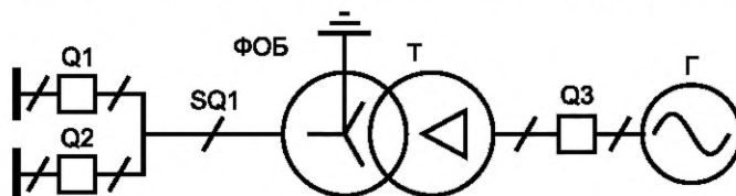
Рисунок А.5 — Тестовая схема 5 для проверки устройств ФОб
