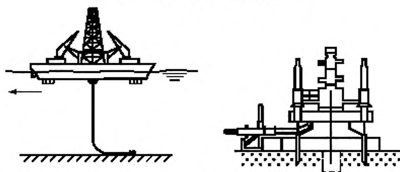
с) Укладка трубы
