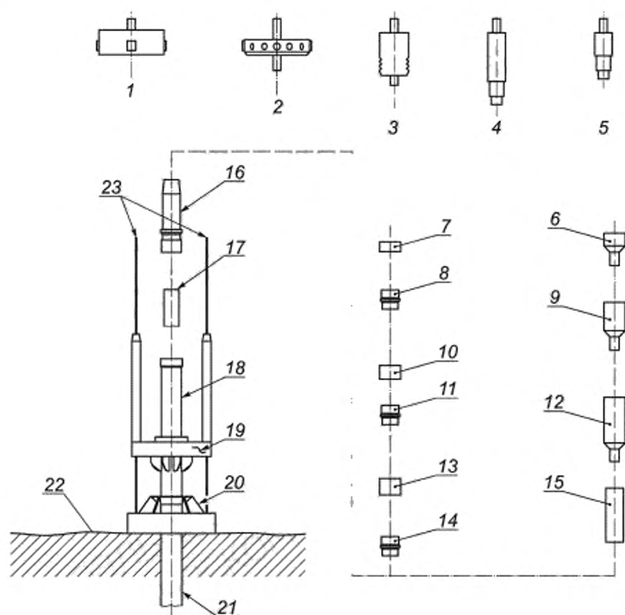
1 — инструмент для установки временной направляющей плиты; 2 — инструмент для установки корпуса направления, 762 мм (30°); 3 — инструмент для установки головки кондуктора; 4 — инструмент для установки ПОК (на буровых или обсадных трубах); 5 — инструмент для испытаний; 6 — защитная втулка, 177,8 мм (7°); 7 — уплотнительный узел межколонного пространства, 244,5 мм на 177,8 мм (9 1/4° на 7°); 8 — ПОК, 177,8 мм (7°); 9 — защитная втулка, 244,5 мм (9 1/4°); 10 — уплотнительный узел межколонного пространства 339,7 мм на 244,5 мм (13 1/4° на 9 1/4°); 11 — ПОК, 244,5 мм (9 1/4°); 12 — защитная втулка, 339,7 мм (13 1/4°); 13 — уплотнительный узел межколонного пространства, 508,0 мм на 339,7 мм (20° на 13 1/4°); 14 — ПОК, 339,7 мм (13 1/4°); 15 — защитная втулка колонной головки; 16 — колонная головка кондуктора; 17 — обсадная колонна, 508,0 мм (20°); 18 — колонная головка направления, рассчитанная на низкое давление, 762,0 мм (30°); 19 — постоянная направляющая плита; 20 — временная направляющая плита; 21 — колонна направления, 762,0 мм (30°); 22 — дно моря; 23 — направляющие
