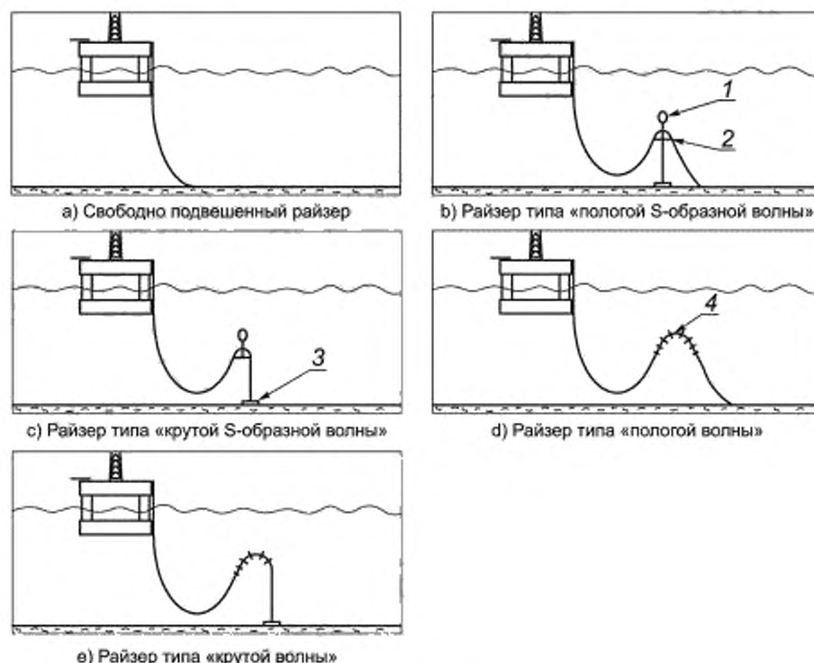
1 — притопленный буй; 2 — направляющее устройство для трубы; 3 — основание райзера; 4 — распределенные элементы, обеспечивающие плавучесть
