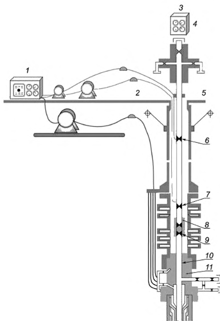
1 — гидравлическая силовая установка и пульт управления; 2 — вертляк (опция); 3 — местный пульт управления; 4 — надводная устьевая арматура; 5 — буровая площадка; 6 — лубрикатор; 7 — запорный клапан; 8 — система аварийного отсоединения; 9 — срезающий клапан; 10 — инструмент спуска трубной головки; 11 — трубная головка
