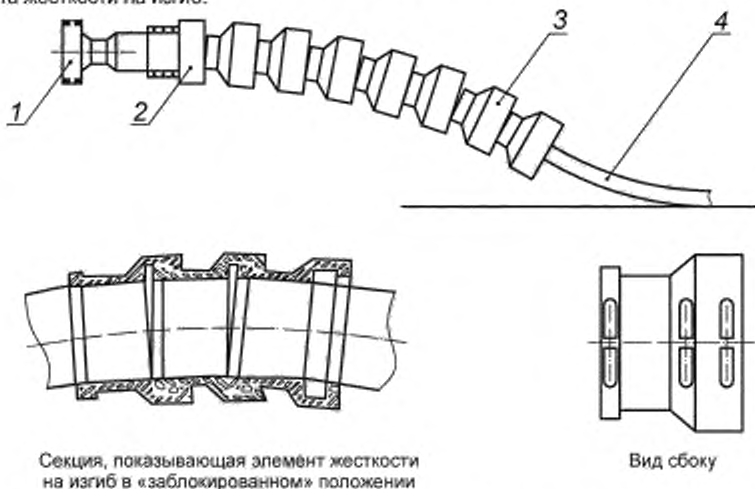
1 — концевой фитинг; 2 — реактивная муфта; 3 — элемент жесткости на изгиб; 4 — подводящая линия
