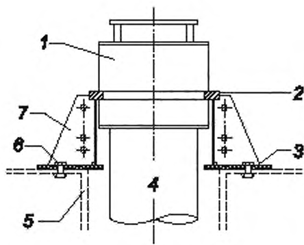
1 — соединительная арматура; 2 — буртик; 3 — фланец; 4 — гибкая труба; 5 — башня; 6 — болты; 7 — хомут
