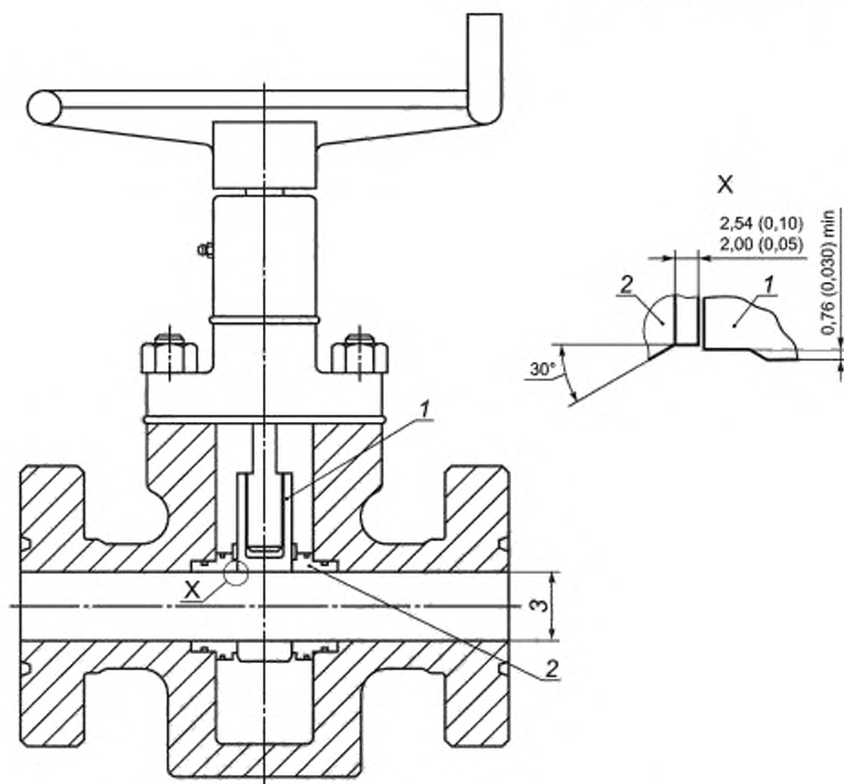
Рисунок 21 — Профили проходных отверстий между заслонкой задвижки и седлом задвижки
