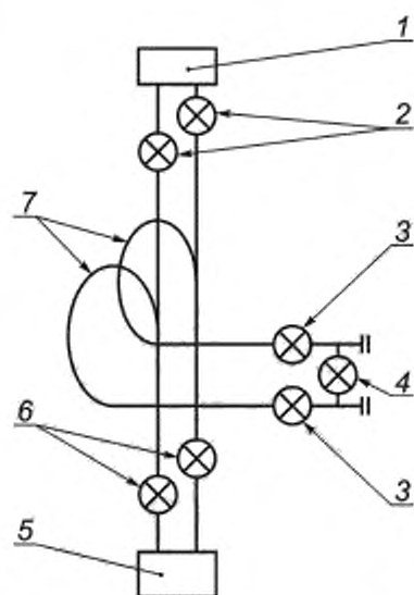
а) Схема типовой фонтанной арматуры системы TFL
