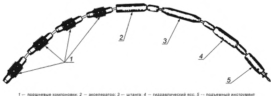
Рисунок 3 — Типовая сервисная колонна системы TFL
