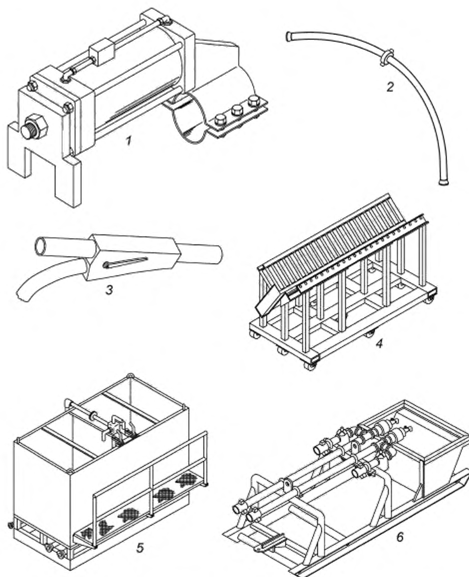
1 — гидравлическое устройство подачи инструмента; 2 — входные трубные петли; 3 — отводные устройства; 4 — ролюганг, 5 — рабочий резервуар, 6 — горизонтальный шлюз
