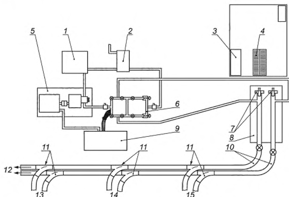
1 — смешительный резервуар для флюидов; 2 — резервуар для хранения; 3 — рабочий стол; 4 — рольганг; 5 — насосный блок; 6 — поверхностный управляющий манифольд; 7 — устройства подачи инструмента; 8 — двойной горизонтальный шлюз; 9 — панель управления; 10 — входные трубные петли; 11 — отводные устройства; 12 — к другим скважинам в системе; 13 — скважина 3; 14 — скважина 2; 15 — скважина 1
