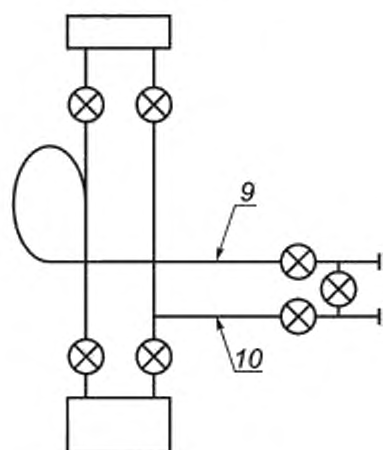
д) «Упрощенная» фонтанная арматура системы TFL
