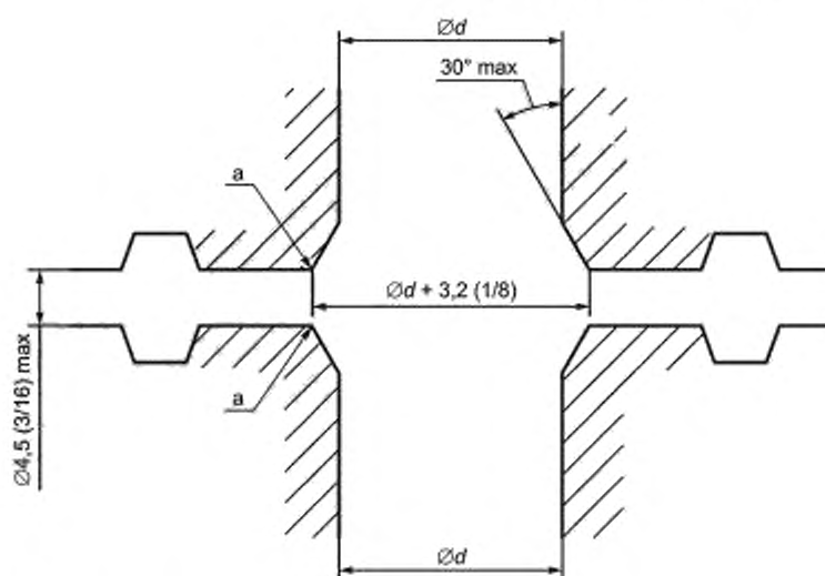
Рисунок 14 — Проточка соединения
