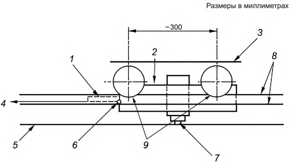
1 — динамометр; 2 — тележка; 3 — платформа; 4 — тяговое устройство; 5 — напольное покрытие; 6 — крепление к тяговому устройству; 7 — ножка; 8 — направляющие рельсы; 9 — ролики
