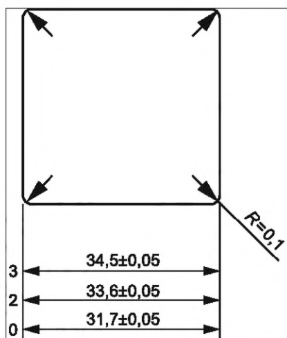
Рисунок 3 — Горизонтальное сечение A-A
