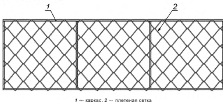
Рисунок 3 — Панель габионной конструкции
