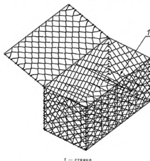
Рисунок 5 — Схема устройства стяжки
