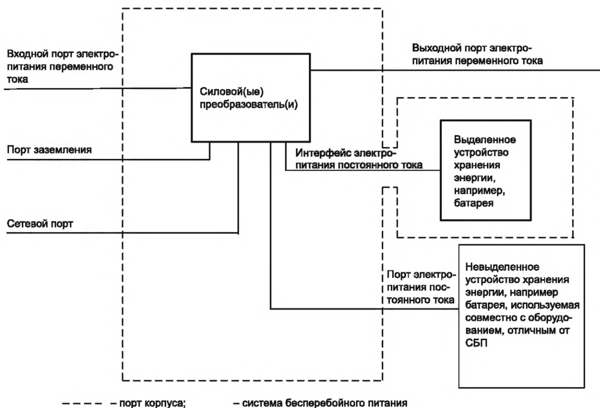
Рисунок 1 — Порты СБП
