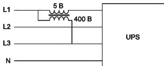
Рисунок D.2 — Фазовая несимметрия
