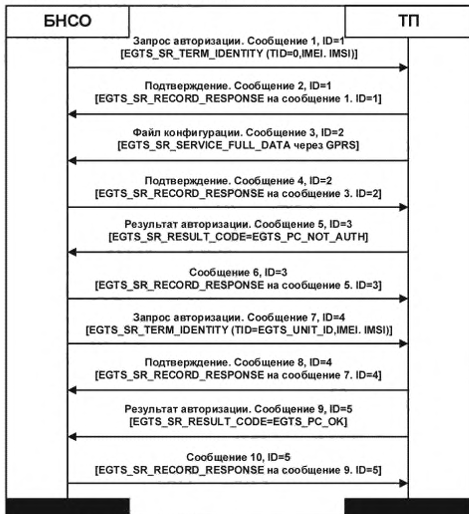
Рисунок Б.3 — Алгоритм обмена сообщениями на этапе авторизации БНКО на ТП
