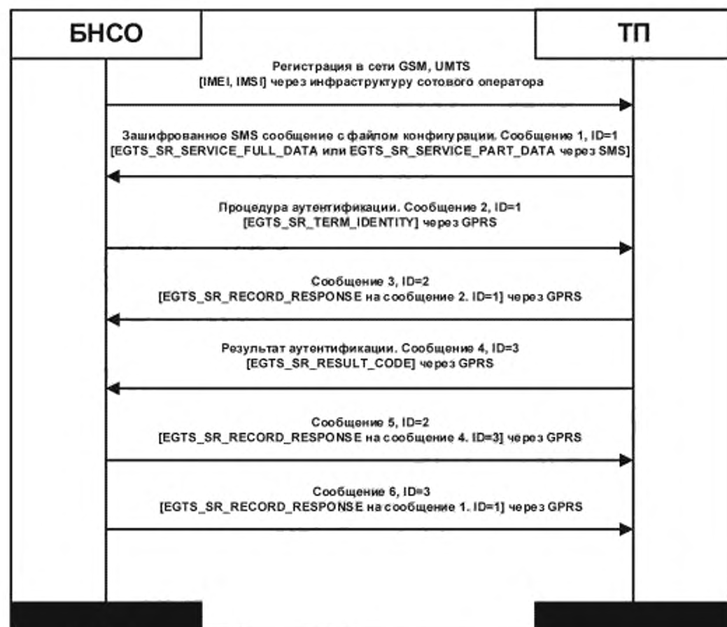
Рисунок Б.1 — Алгоритм конфигурации BHCO с использованием SMS
