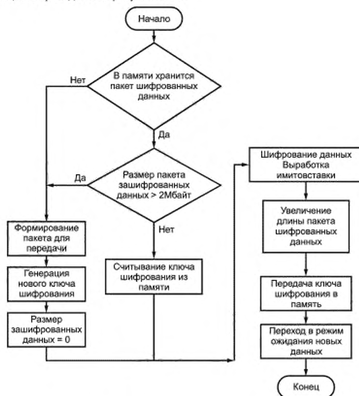
Рисунок 3 — Схема передачи данных от БНСО на сервер
