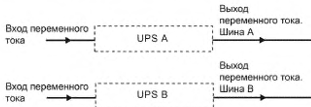
Рисунок A.6 — UPS с двумя шинами
