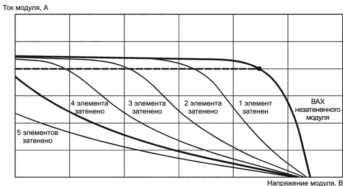
Рисунок 7 — Пример ВАХ монолитного тонкопленочного модуля с последовательным соединением фотоэлектрических элементов при затенении разного количества элементов
