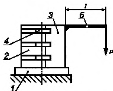
Рисунок 1 — Схема приложения испытательной силы к консольной части аппарата
