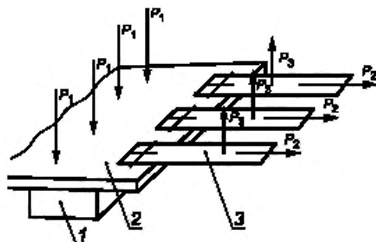
1 — стол испытательного устройства; 2 — испытуемый образец аппарата (гильза, корсет, полукорсет или пояс); 3 — элементы текстильной застежки; P_1 — сила прижима; P_2 — испытательная сила; P_3 — сила отрыва
