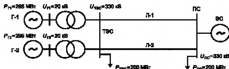
Г-1, Г-2 — генератор 1 и 2; Л-1, Л-2 — линия электропередачи 1 и 2; ЭС — энергосистема; P_{TSC} — нагрузка в узле ТЭС; P_{PC} — нагрузка в узле ПС; P_{G1} , P_{G2} — активная мощность генератора 1 и 2; U_{G1} , U_{G2} — номинальное напряжение генератора 1 и 2; U_{PC} — напряжение в узле ПС; U_{TSC} — напряжение в узле ТЭС
