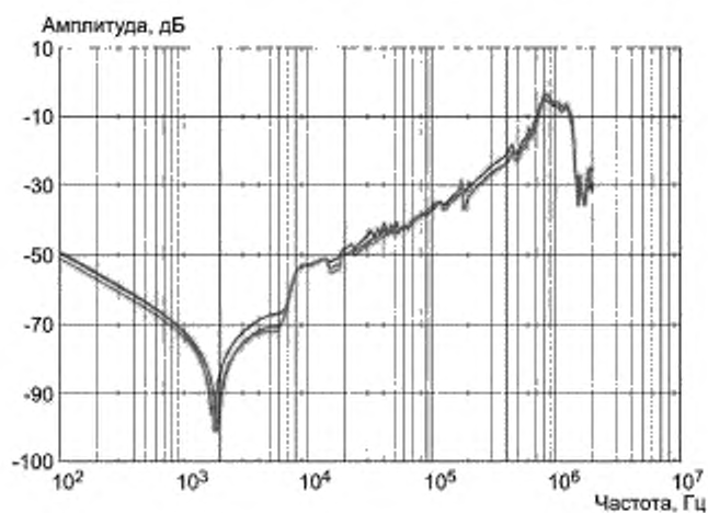
Рисунок А.4 — Сравнение с частотными характеристиками одностипных трансформаторов
