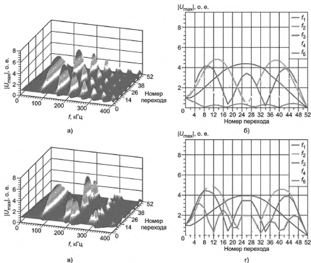
Рисунок ДА.3 — Спектральные распределения напряжений а), в) и распределения напряжений на первых пяти собственных частотах ( f_1, f_2, f_3, f_4 и f_5 соответственно) обмотки б), г) в катушечной обмотке без замыканий а), б) и при замыкании катушек в середине высоты в), г)
