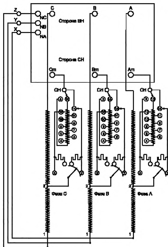
A, B и C — выводы стороны BH ; Am, Bm и Cm — выводы стороны CH ; X, Y и Z — выводы концов общей обмотки; NA, NB и NC — выводы нейтрали (отдельные выводы для каждой из трех фаз)
