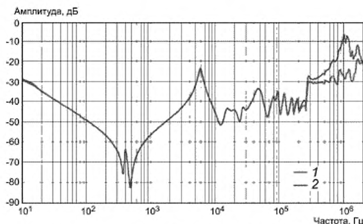
1 — измерение от линейного вывода к нейтрали обмотки ВН; 2 — измерение от нейтрали к линейному выводу обмотки ВН
