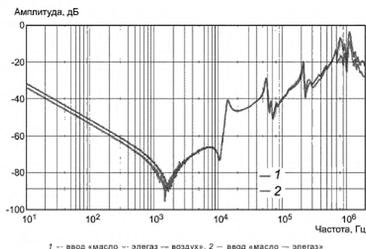
Рисунок А.15 — Влияние высоковольтного ввода на частотные характеристики
