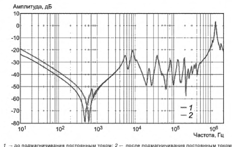
Рисунок А.14 — Влияние остаточной намагненности на частотные характеристики
