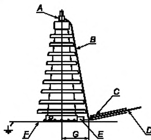
А — соединительный зажим; В — плетёный проводник или провод минимальной длины; С — экран измерительного кабеля; D — центральный проводник кабеля; E — зажим заземления; F — бак трансформатора (реактора); G — кратчайшая петля
