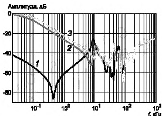
1 — обмотки НН1 и НН2 разомкнуты; 2 — обмотка НН1 замкнута, 3 — обмотки НН1 и НН2 замкнуты
