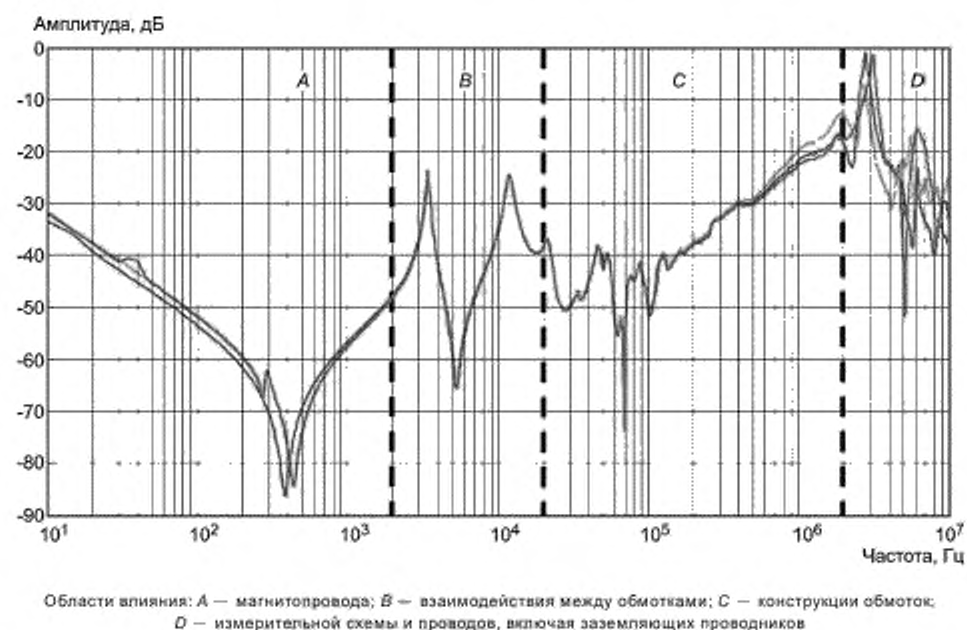
Рисунок А.6 — Частотная характеристика и области влияния конструктивных элементов трансформатора и схемы измерений на примере последовательной обмотки автотрансформатора
