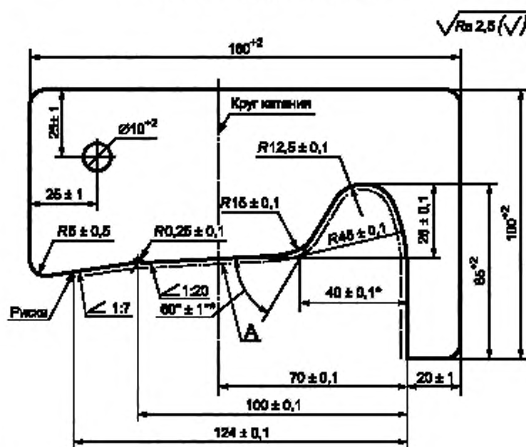
Рисунок А.1 — Профиль обода колеса
