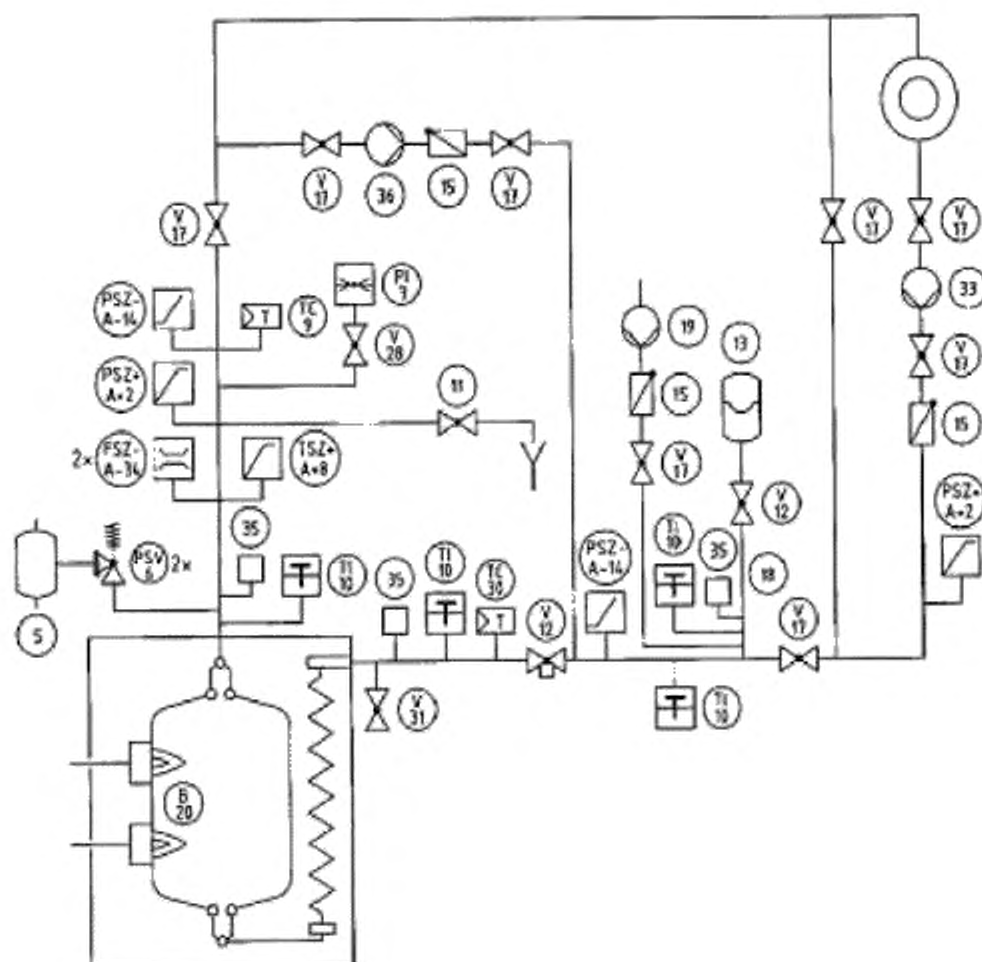
Рисунок В.4-10 — Установки с принудительной циркуляцией, поддержанием давления из внешнего источника, газовым аккумулятором и наложенной рециркуляцией
