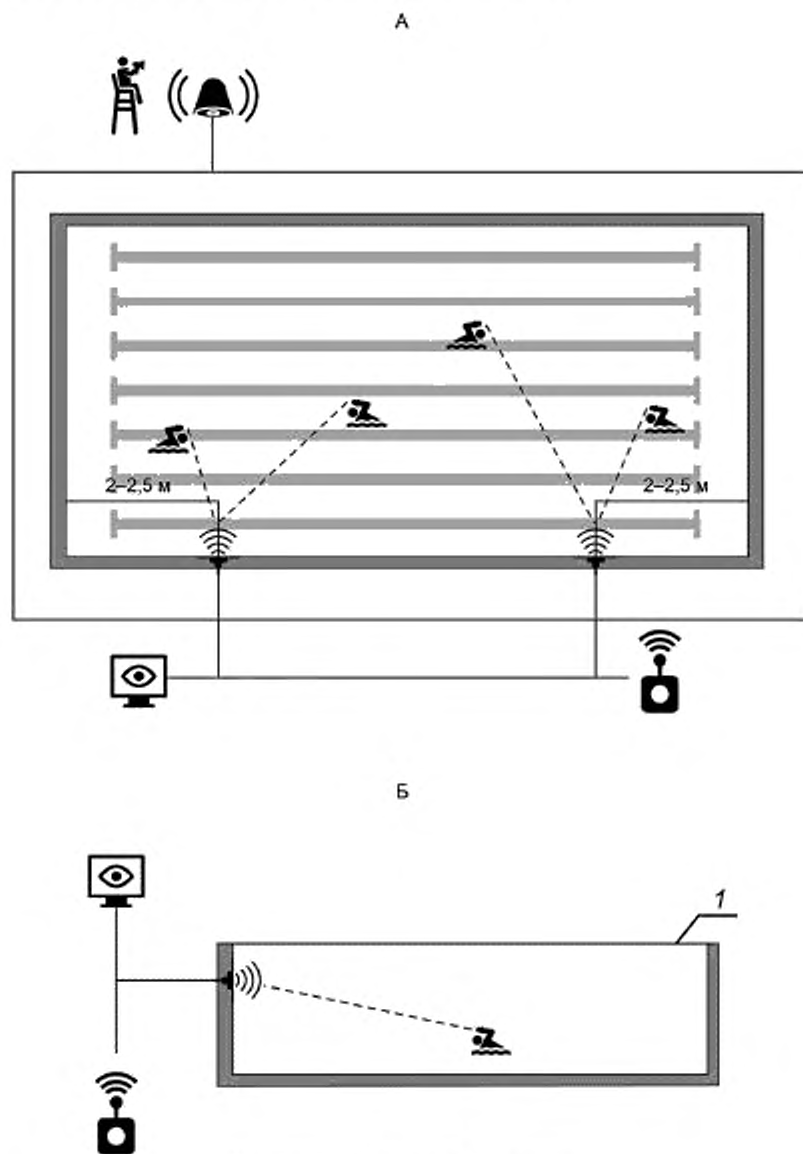
Рисунок Б.1 — Размещение компонентов системы УзСОУ
