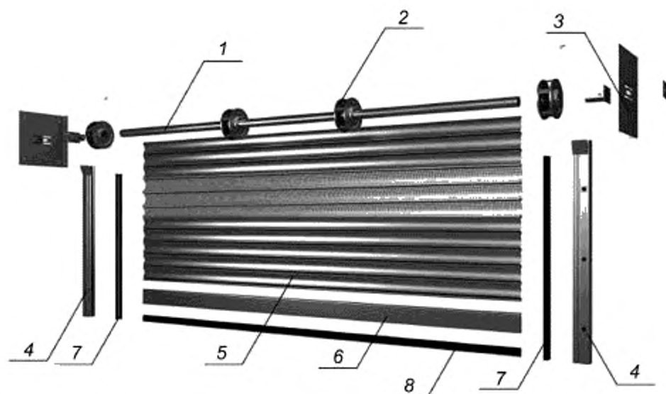
1 — намоточный вал, 2 — барабанный ПИМ; 3 — консольный кронштейн, 4 — направляющие (шины); 5 — роллетное полотно; 6 — концевой профиль; 7 — боковой уплотнитель; 8 — нижний уплотнитель
