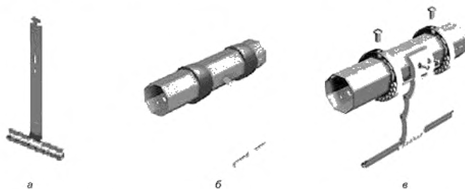
а — тяговая пружина; б — тяговая пружина, закрепленная на валу с помощью ригельных колец, в — блокирующий подвес, закрепленный на валу с помощью ригельных колец
