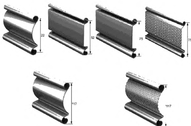
Рисунок Г.1 — Одностенные стальные профили роликовой прокатки
