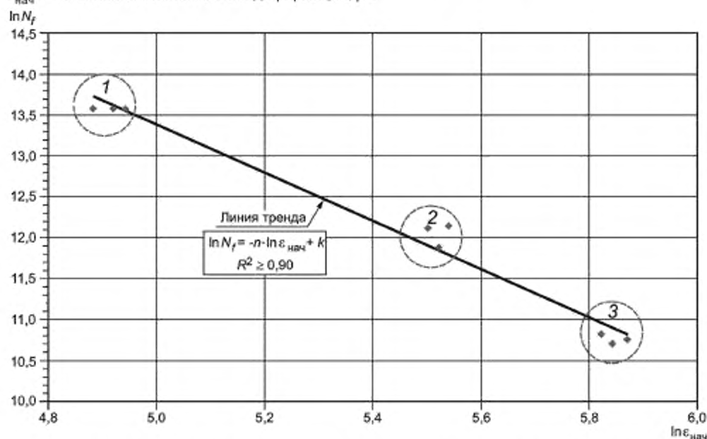
Рисунок 5 — Пример корреляционной зависимости между логарифмом относительной начальной деформации и логарифмом количества циклов нагружения
