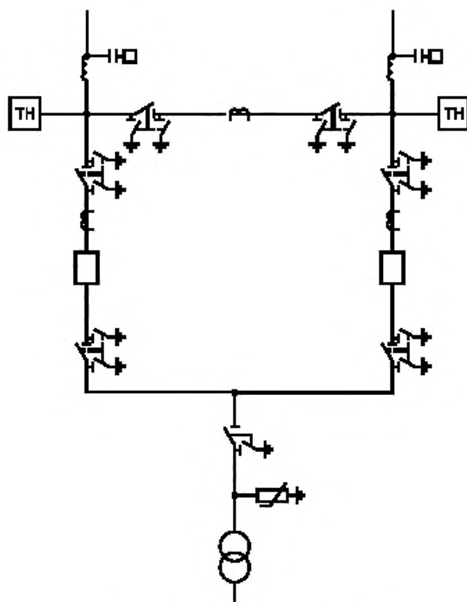
Рисунок 29 — Схема 220-6. «Заход—выход»
