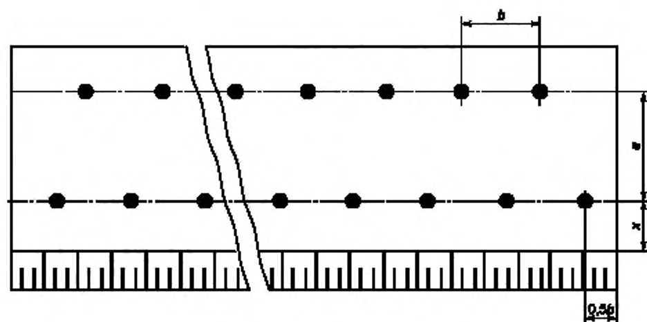
Рисунок 2 — Двухрядное расположение скважин
