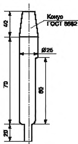
Рисунок 2 — Кварцевая вставка
