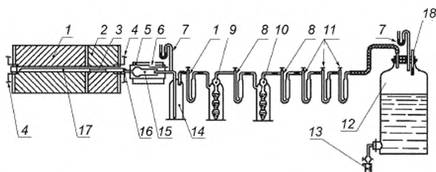
1 — электрическая трубчатая печь для коксования; 2 — электрическая трубчатая печь для пиролиза; 3 — насадки из четырех рядов фарфоровых бусинок; 4 — одноточечные и пятиточечные термопреобразователи; 5 — электрическая трубчатая печь для кварцевой трубки с ватным фильтром; 6 — термометр или термопреобразователь; 7 — жидкостной мановакуумметр; 8 — U-образные трубки с хлористым кальцием; 9 — поглотительная склянка для диоксида углерода и сероводорода; 10 — поглотительная склянка для непредельных углеводородов; 11 — U-образные трубки с активным углем; 12 — склянка для сбора газа (газометр); 13 — мерный цилиндр; 14 — поглотительная склянка для аммиака; 15 — кварцевая трубка с ватным фильтром для улавливания смолы; 16 — кварцевая вставка; 17 — реакционная кварцевая трубка; 18 — термометр
