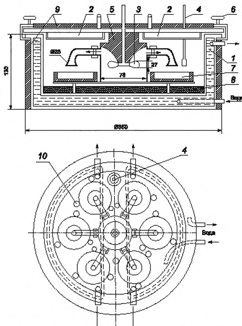
Рисунок 1 — Аппарат для кондиционирования
