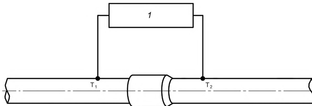
Рисунок В.1 — Схема измерений «кажущегося» сопротивления для трубопроводов надземного и подземного размещения
