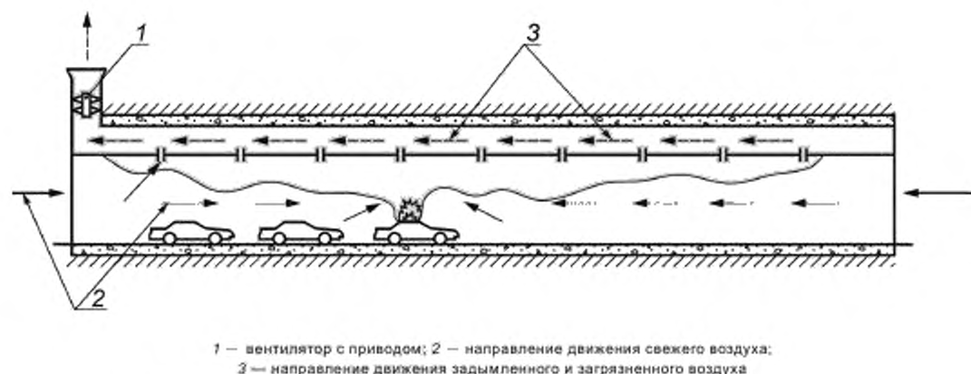
Рисунок 12.3 — Противодымная защита с продольно-поперечной схемой вентиляции
