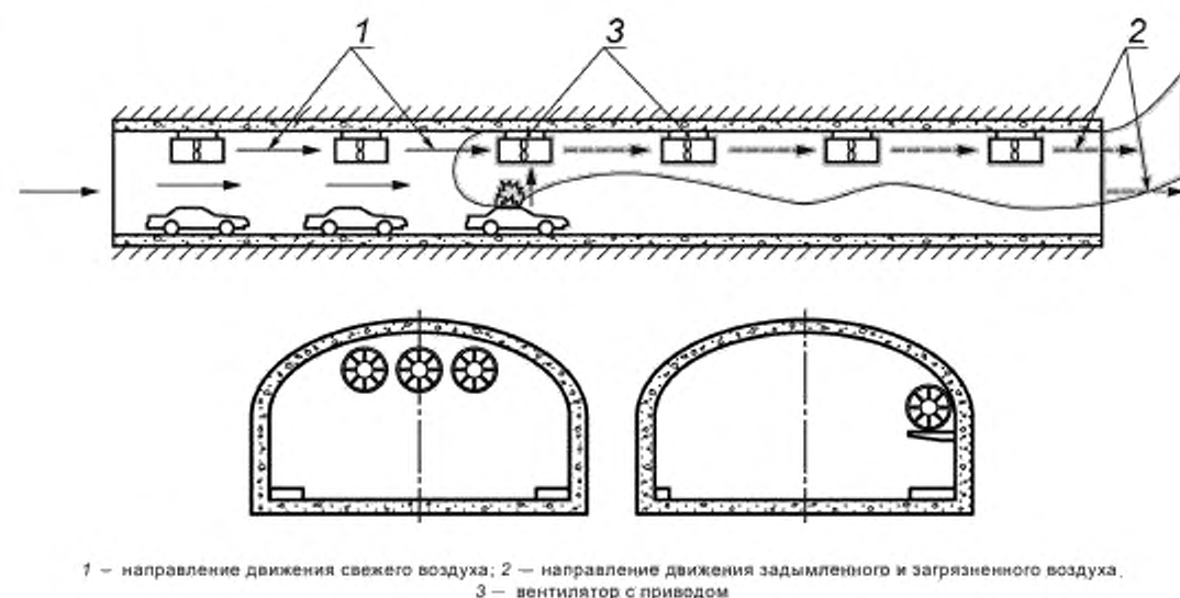
Рисунок 12.1 — Противодымная защита с продольной схемой вентиляции и применением струйных вентиляторов
