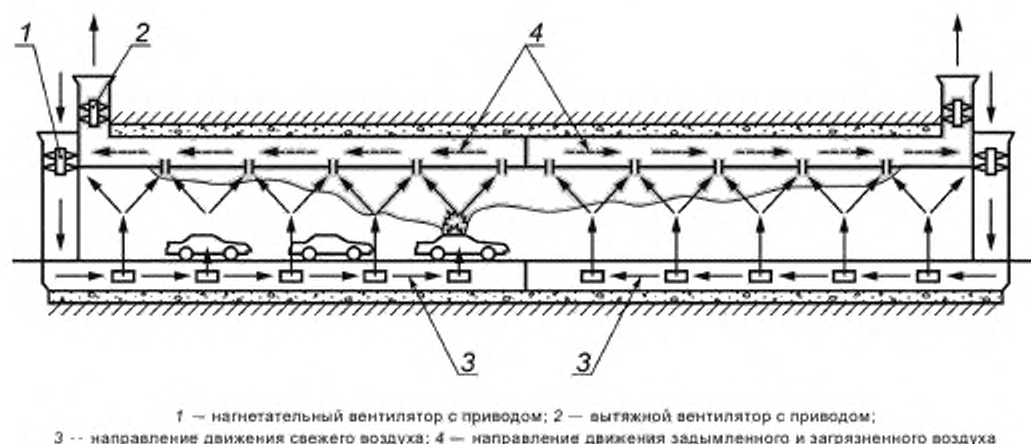
Рисунок 12.2 — Противодымная защита с поперечной схемой вентиляции
