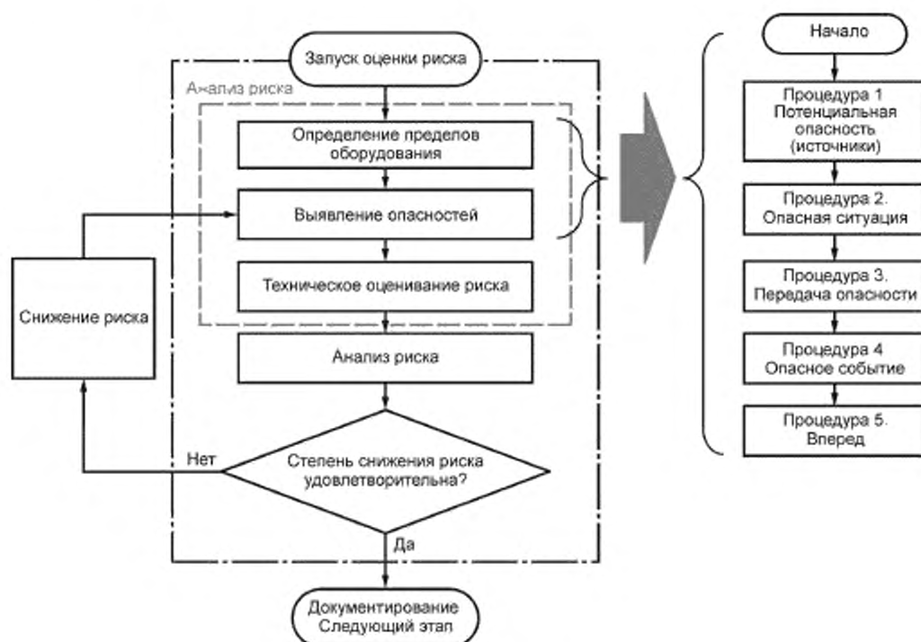
Рисунок С.1 — Метод оценки риска
