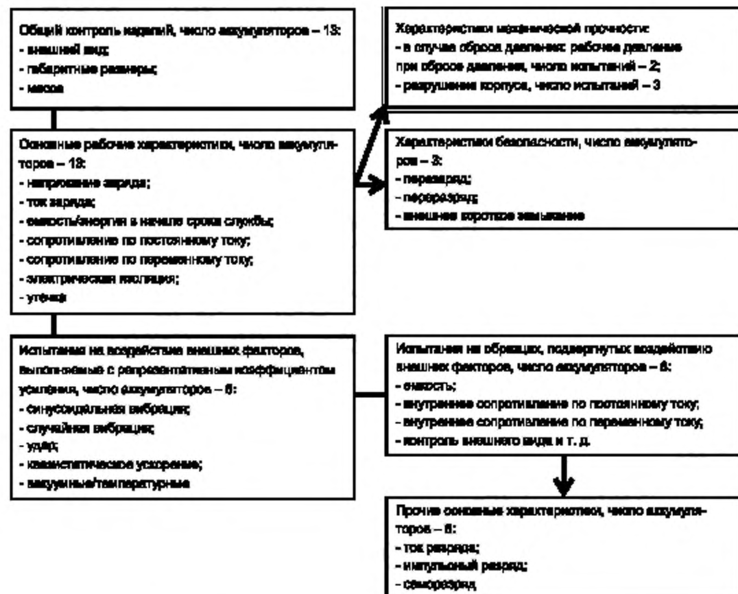
Рисунок В.1 — Порядок проведения квалификационных испытаний
