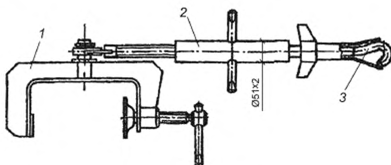
1 — струбина, 2 — винтовой механизм; 3 — крюк
