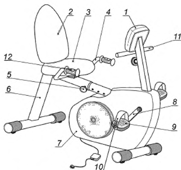
1 — дисплей; 2 — спинка сиденья; 3 — сиденье; 4 — рукоятки сиденья; 5 — регулятор сиденья; 6 — рама; 7 — защитный кожух; 8 — кривошип; 9 — педаль; 10 — ремень педали; 11 — передние рукоятки; 12 — наружный датчик пульса
