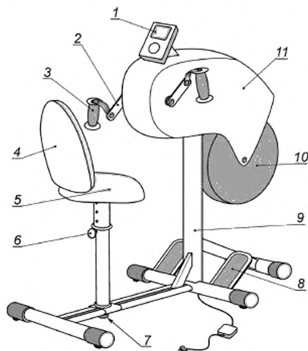
1 — дисплей; 2 — кривошип; 3 — ручка; 4 — спинка сиденья; 5 — сиденье; 6 — регулятор положения сиденья по вертикали; 7 — регулятор положения сиденья по горизонтали; 8 — упор для ног; 9 — рама; 10 — маховик; 11 — защитный кожух
