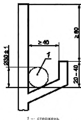
Рисунок 1 — Размеры опоры штанги
