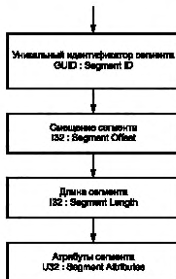
Рисунок 5 — Данные записи содержания файла
