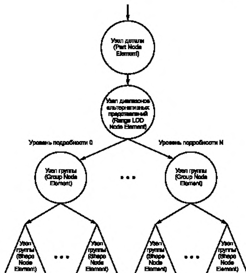
Рисунок 6 — Иерархия узлов модели при описании детали в общей структуре модели
