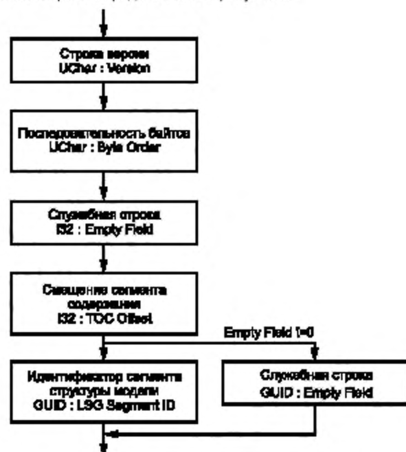
Рисунок 3 — Данные сегмента заголовка файла
