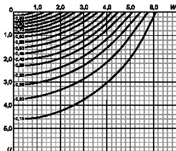
Рисунок В.11 — Графики значений при a_2 = \frac{\sigma_2}{p_0} \frac{2a}{B} = 6
