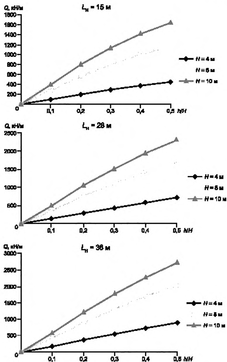
Рисунок 9 — Расчетные графики гидростатического всплытия насыпи с заложением откоса 1:1,5 при коэффициенте запаса 1,1, при трех вариантах ширины дороги
