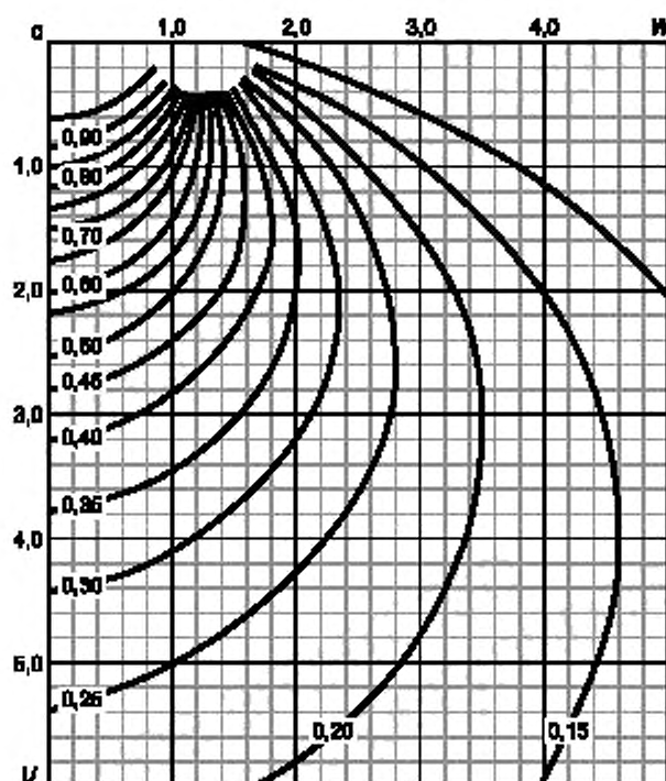
Рисунок В.2 — Графики значений при a_1 = \frac{\sigma_1}{\rho_0} \frac{2a}{B} = 0,2
