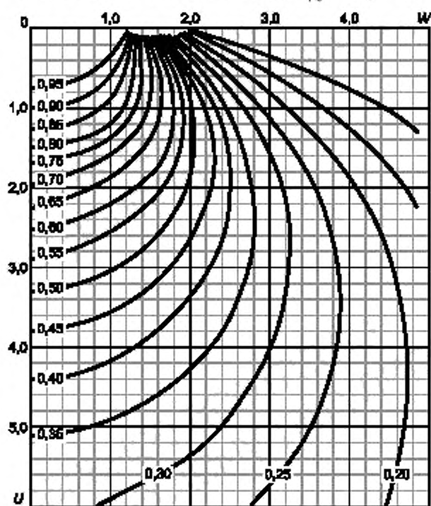
Рисунок В.4 — Графики значений при a_1 = \frac{\sigma_1}{\rho_0} \frac{2a}{B} = 1
