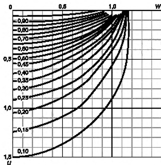
Рисунок В.3 — Графики значений при a_2 = \frac{\sigma_2}{\rho_0} \frac{2a}{B} = 0,2
