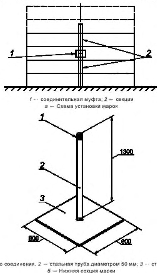
Рисунок 15 — Схема установки осадочных марок
