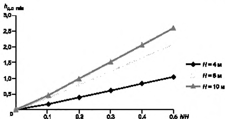
Рисунок 7 — Графическая зависимость минимальной толщины дорожной одежды h_{д.о. min} при коэффициенте запаса по всплытию 1,1 от отношения уровня воды к высоте насыпи h/H
