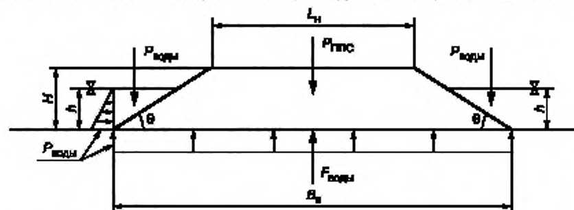
H — высота насыпи, м; h — уровень воды, м; L_n — ширина насыпи поверху, м; B_n — ширина насыпи понизу, м; F_{воды} — подъемная сила воды, кН/м; P_{ппс} — вес насыпи из ППС блоков, кН/м; P_{воды} — удерживающая сила воды, действующая на откосы, кН/м; \theta — угол заложения откоса, градусы; R_{воды} — давление воды, оказываемое на основание и поверхности откосов насыпи, кН
