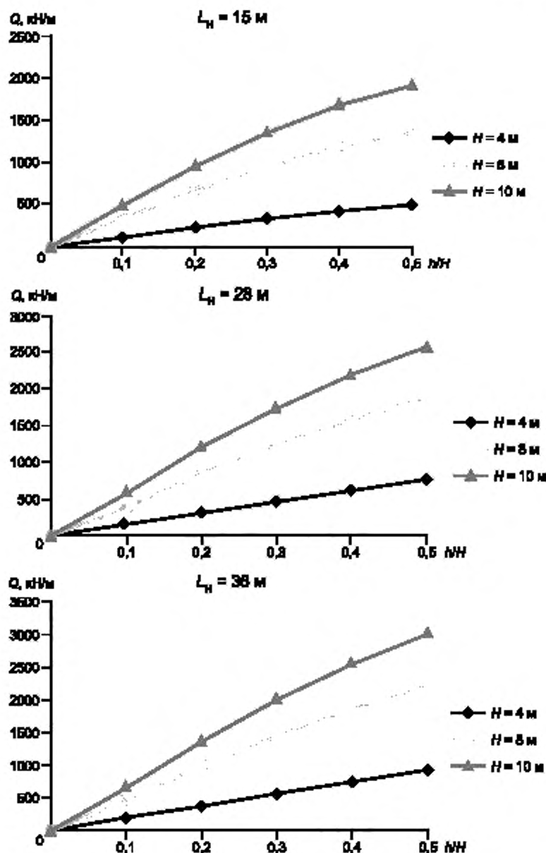
Рисунок 11 — Расчетные графики гидростатического всплывания насыпи с заложением откоса 1:2 при коэффициенте запаса 1,1, при трех вариантах ширины дороги
