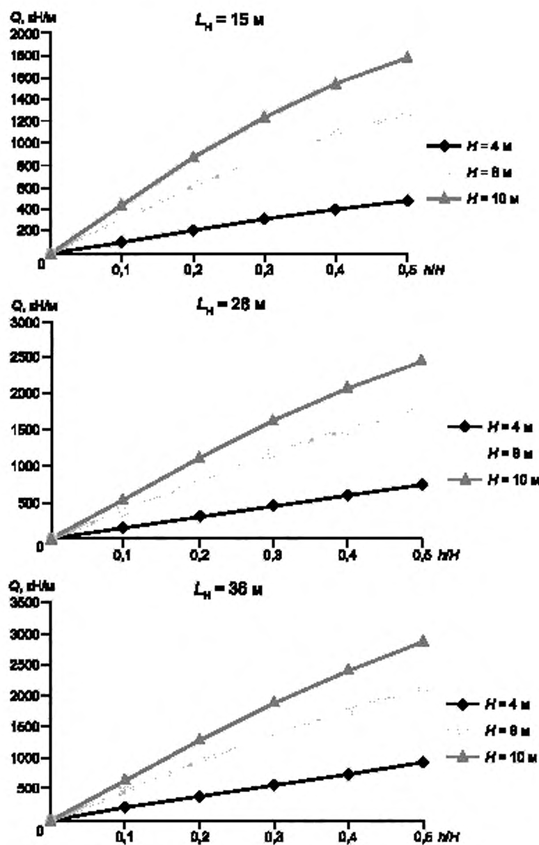
Рисунок 10 — Расчетные графики гидростатического всплытия насыпи с заложением откоса 1:1,75 при коэффициенте запаса 1,1, при трех вариантах ширины дороги
