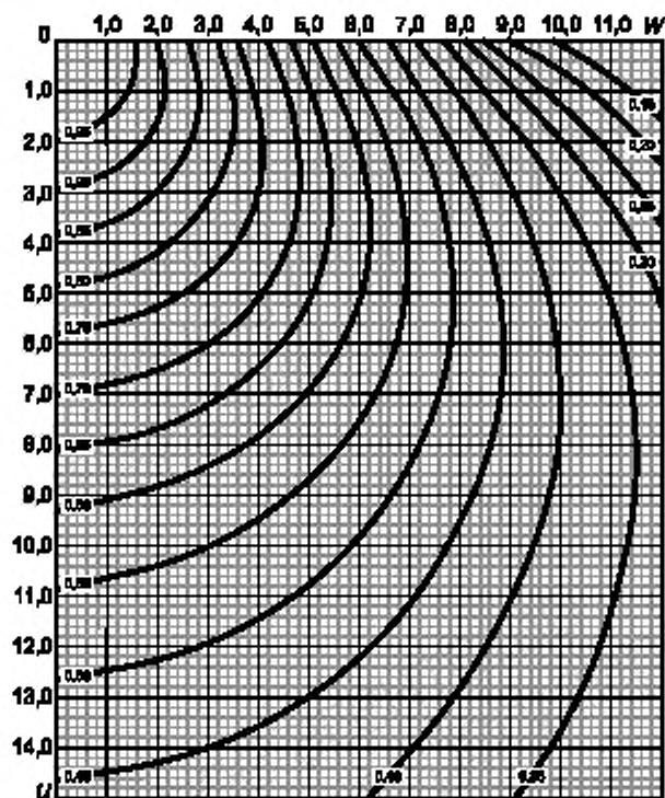
Рисунок В.12 — Графики значений при a_1 = \frac{\sigma_1}{p_0} \frac{2a}{B} = 10
