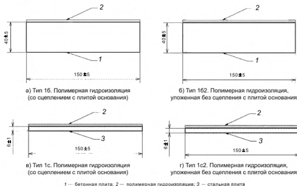
Рисунок 1 — Испытуемые образцы типов 16, 1с, 162 и 1с2
