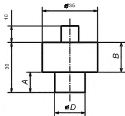
A — высота наконечника; B — высота оправы; D — диаметр наконечника
