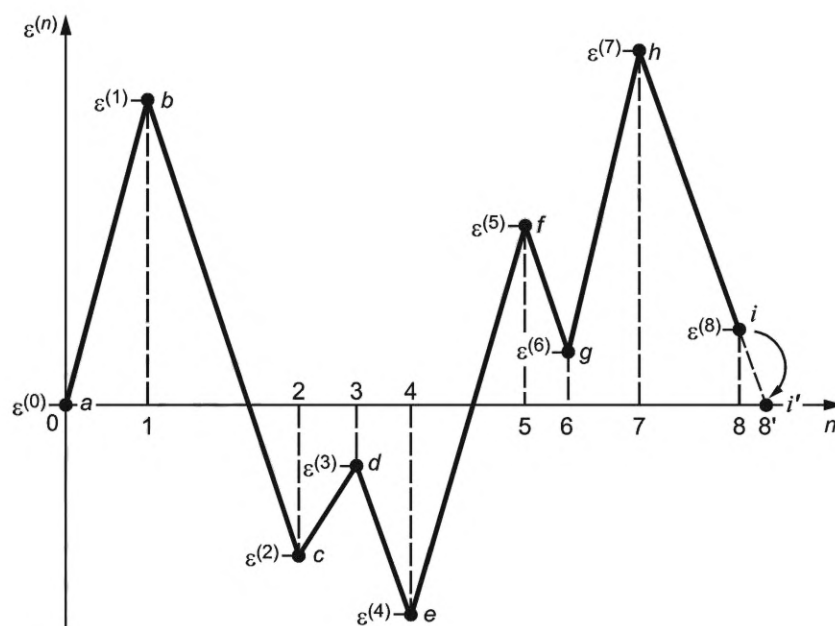
Рисунок Ж.2 — Зависимость \varepsilon(n) от номера шага нагружения и применение метода «стока» для определения размахов деформаций \Delta\varepsilon , цикла (полуцикла) N с размахом деформаций \Delta\varepsilon и при общем количестве циклов нагружения K = 6
