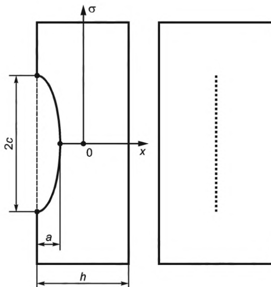
Рисунок К.1 — Полуэллиптическая поверхностная трещина
