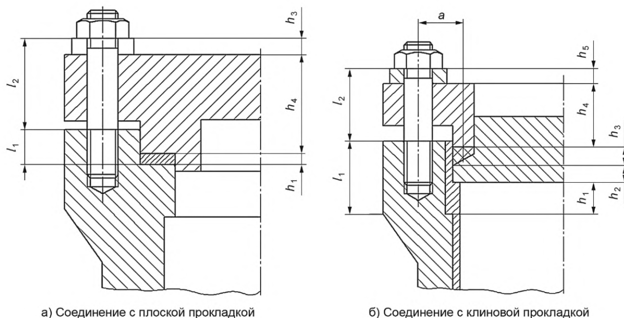
Рисунок 4.1 — Типовые конструкции разъёмных соединений
