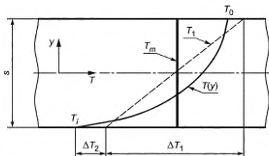
Рисунок 6.4 — Расчетные размахи температур по толщине стенки
