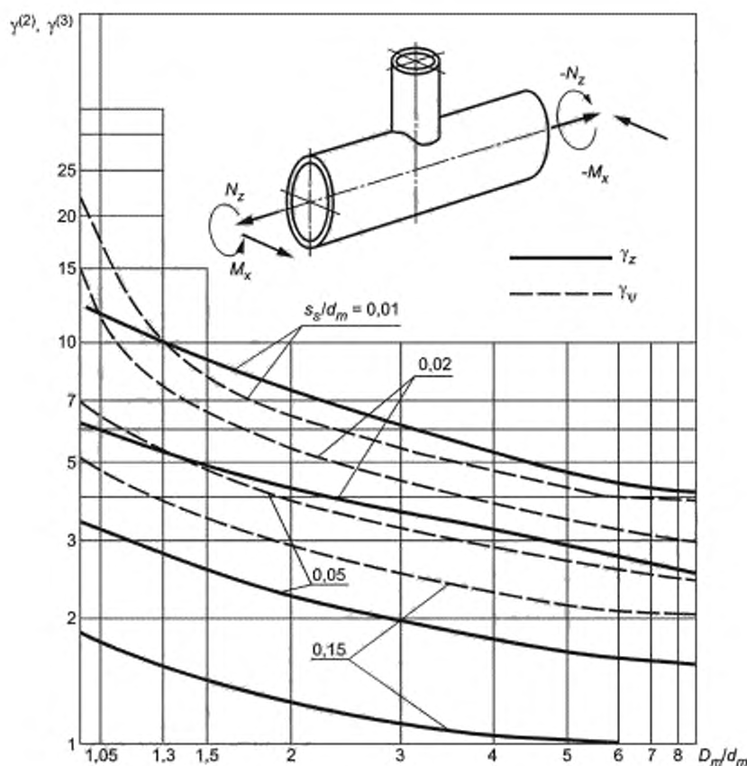
Рисунок А.10 — Номограммы для определения коэффициентов \gamma^{(2)} и \gamma^{(3)}
