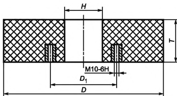
Рисунок 11 — Круги типа 36
