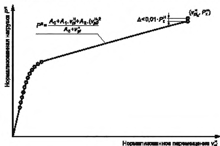
Рисунок K.4 — Аппроксимация нормализованной диаграммы уравнением (K.7)
