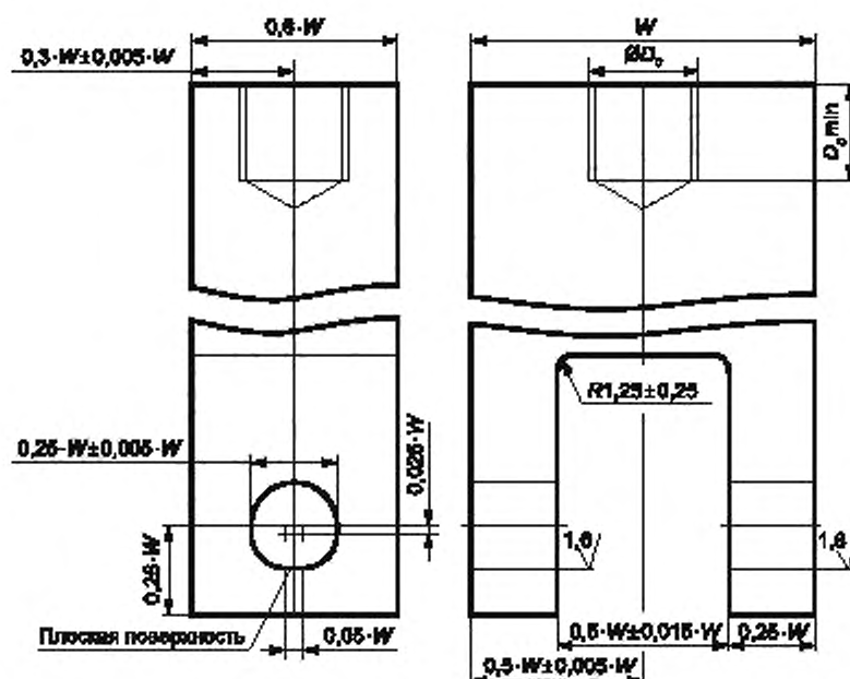
Рисунок 7.1 — Захват (вилка) для установки образцов типов CT, DT
