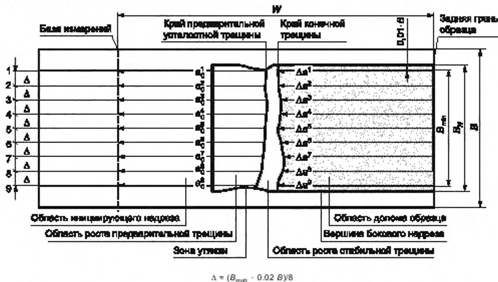
Рисунок Ж.1 — Схема определения длины предварительной усталостной трещины и величины стабильного подроста трещины для образцов типов CT, SE(B) и DT
