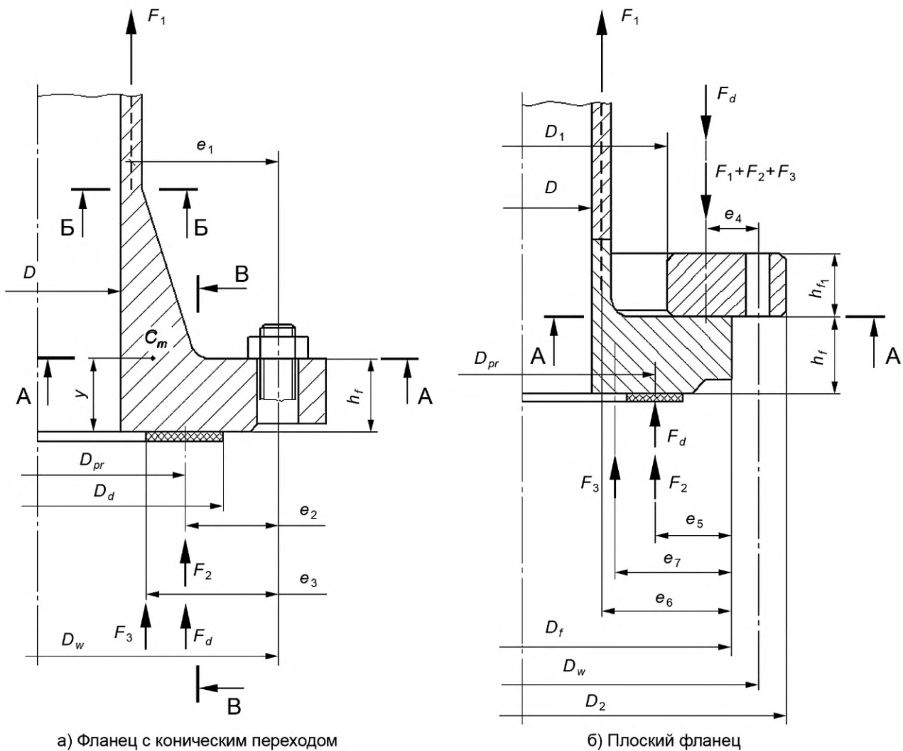
Рисунок В.2 — Расчетная схема фланцев
