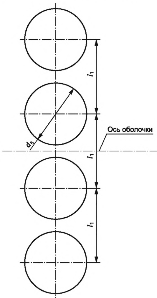
Рисунок 6.8 — Поперечный ряд отверстий с одинаковым шагом
