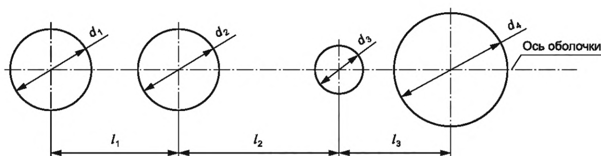
Рисунок 6.11 — Ряд отверстий с неодинаковыми отверстиями и шагами
