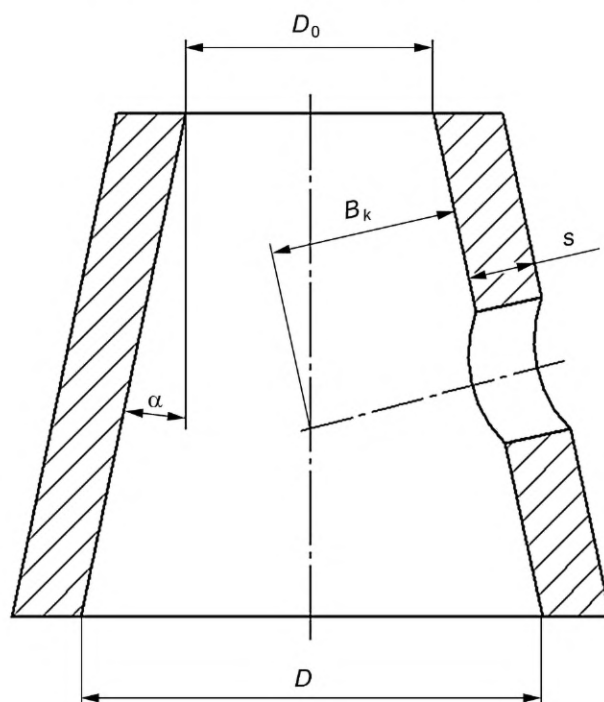
Рисунок 5.2 — Коническая обечайка
