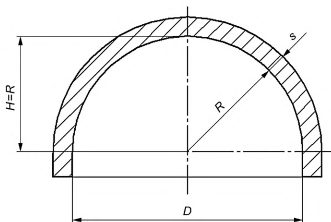
Рисунок 5.4 — Полусферическое днище
