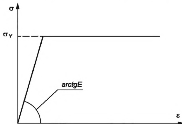
Рисунок А.1 — Диаграмма растяжения идеального упругопластического материала
