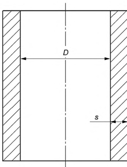
Рисунок 5.1 — Цилиндрическая обечайка
