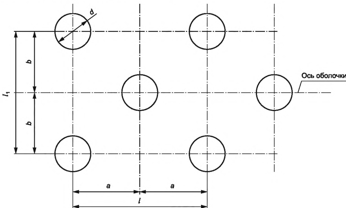
Рисунок 6.9 — Шахматное расположение отверстий
