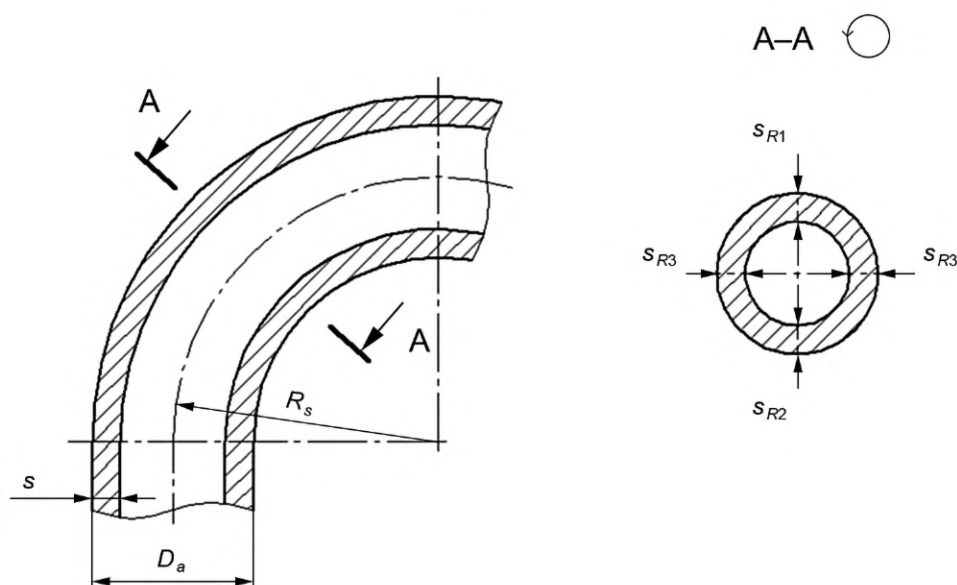
Рисунок 5.5 — Отвод
