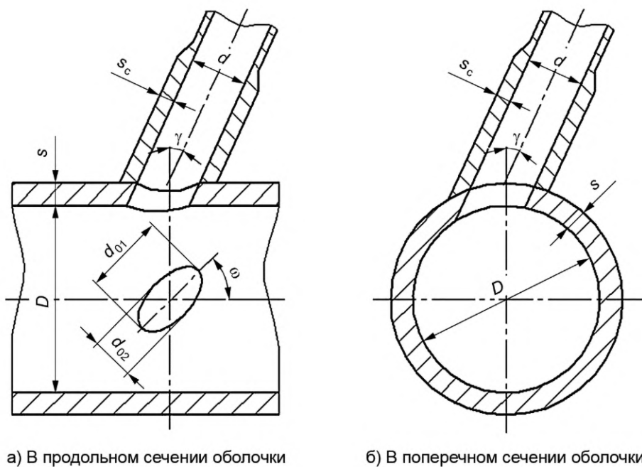
Рисунок 6.5 — Наклонные штуцеры
