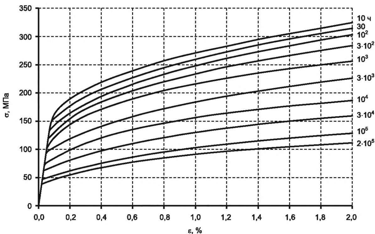
а) При T = 773 \text{ К (} 500 \text{ °C)}
