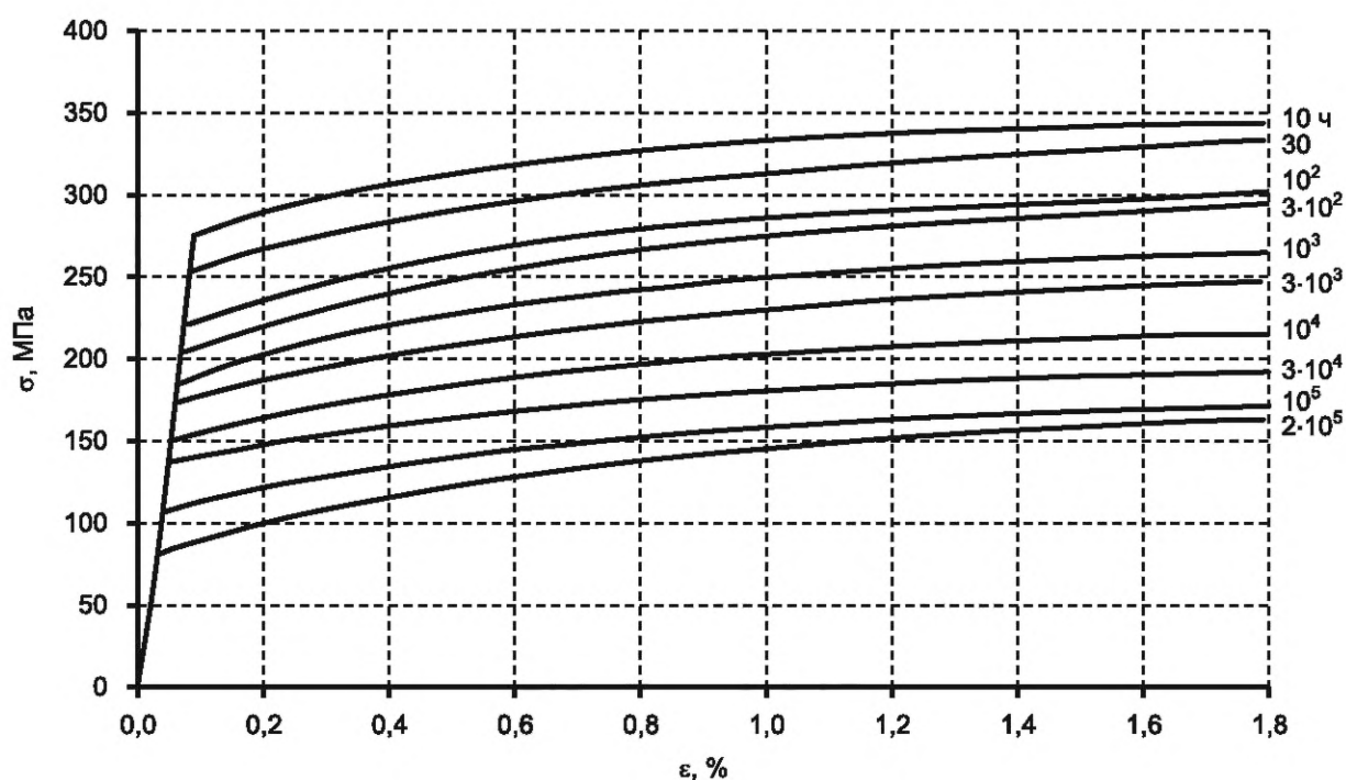
Рисунок Б.7 — Изохронные кривые деформирования стали марки 05X12H2M ( R_{\rho 0,2}^{20} = 372 \text{ МПа} ; R_m^{20} = 539 \text{ МПа} )
