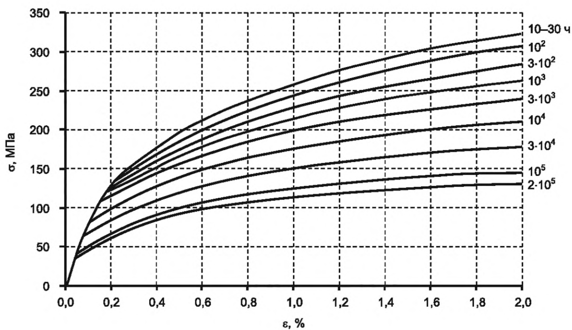
Рисунок Б.6 — Изохронные кривые деформирования стали марки 12X1МФ ( R_{p0,2}^{20} = 274 \text{ МПа} ; R_m^{20} = 441 \text{ МПа} )
