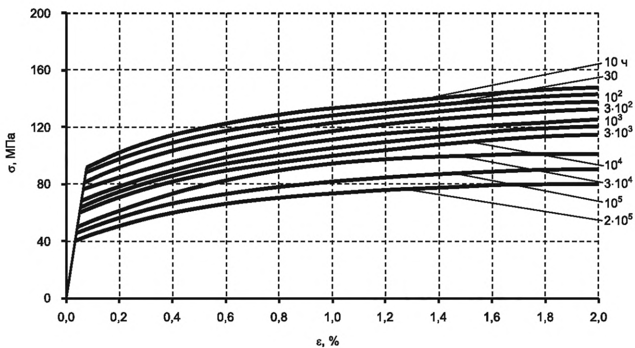
г) При T = 873 \text{ K} ( 600^\circ\text{C} )
