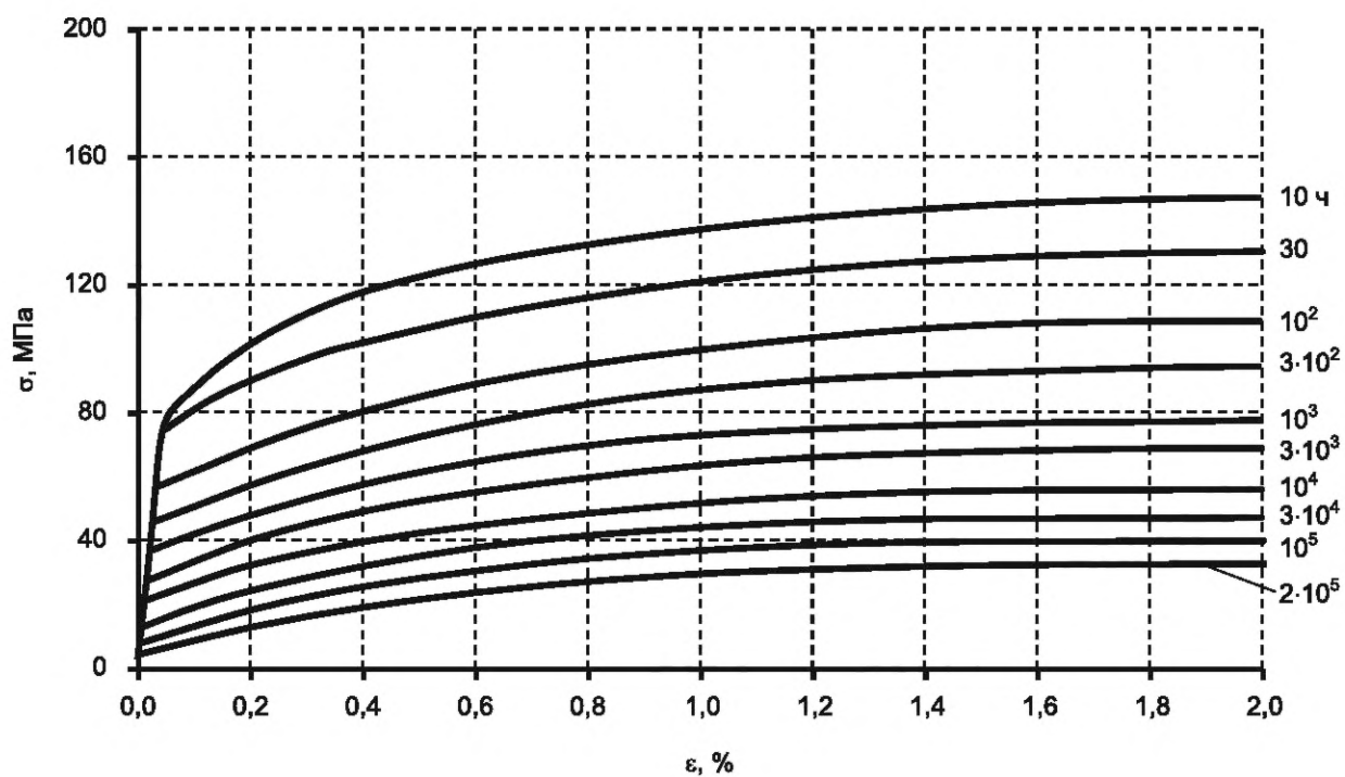
г) При T = 570^\circ\text{C}
