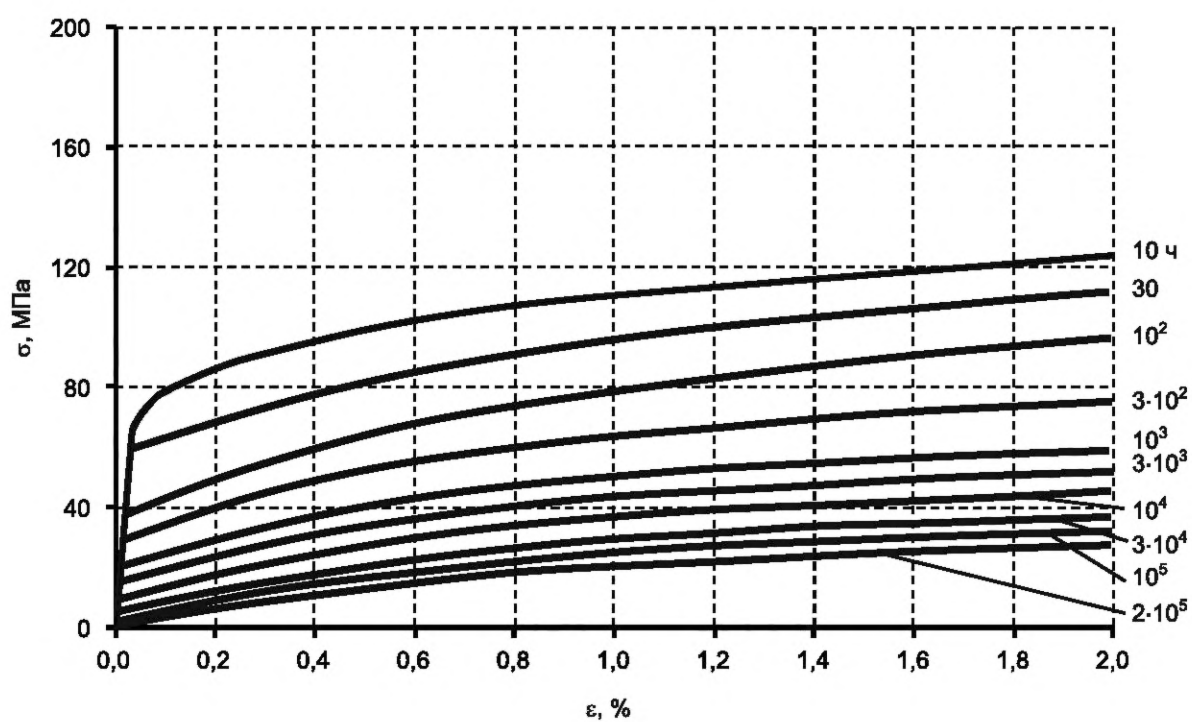
д) При T = 873 \text{ K} ( 600 \text{ °C} )
