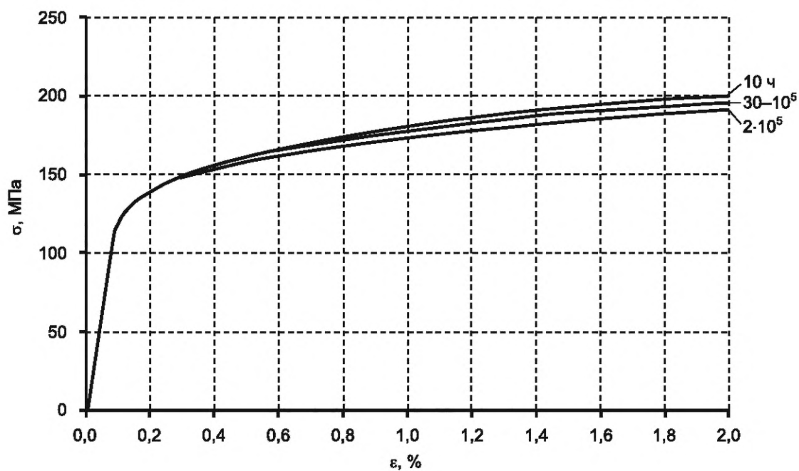
Рисунок Б.4 — Изохронные кривые деформирования стали марки 12X18H9 ( R_{p0,2}^{20} = 196 \text{ МПа} ; R_m^{20} = 490 \text{ МПа} )
