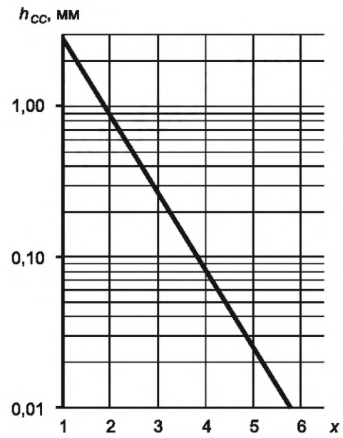
Рисунок Д.4 — Диаграмма науглероживания стали марки 12X16H15M3Б в жидком натрии, x = \frac{6050}{T} - \lg t ( T , К)
