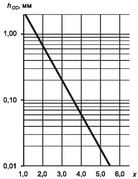
Рисунок Д.3 — Диаграмма науглероживания сталей марок 09X18H9, 10X18H9, 12X18H9, 08X16H11M3, 12X18H10T в жидком натрии, x = \frac{6050}{T} - \lg t ( T , К)
