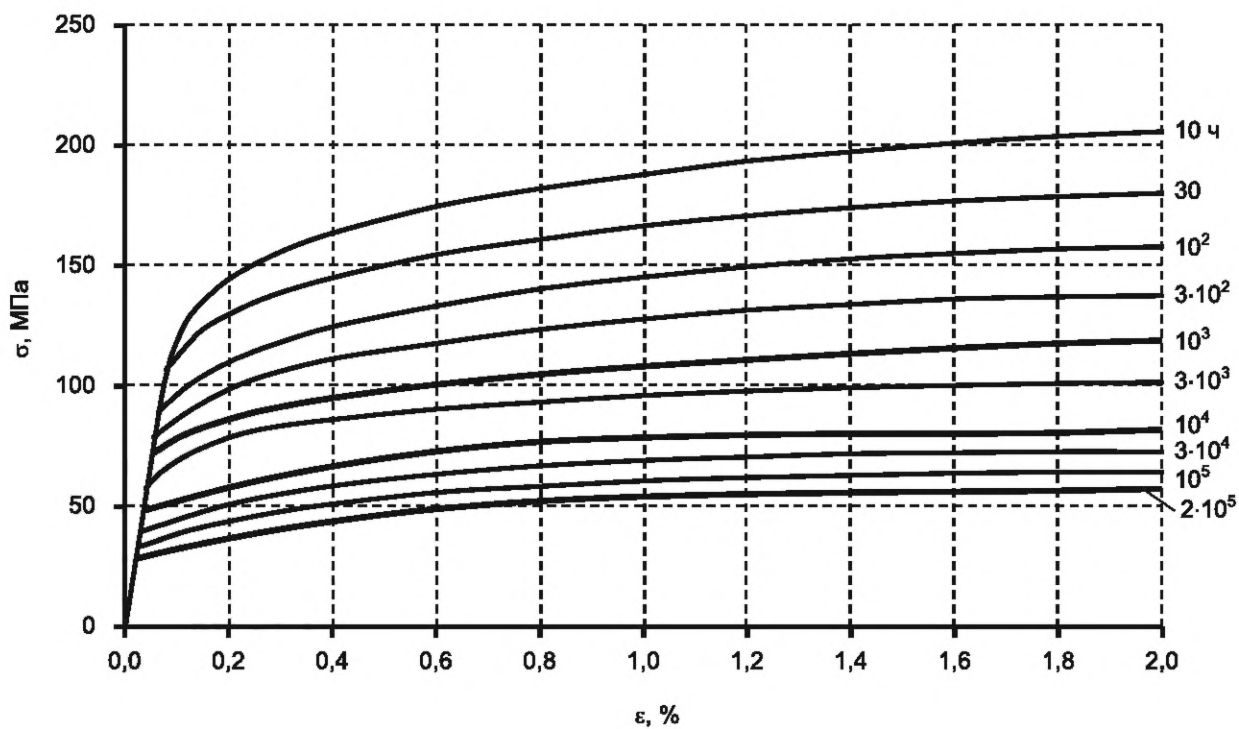
в) При T = 550^\circ\text{C}
