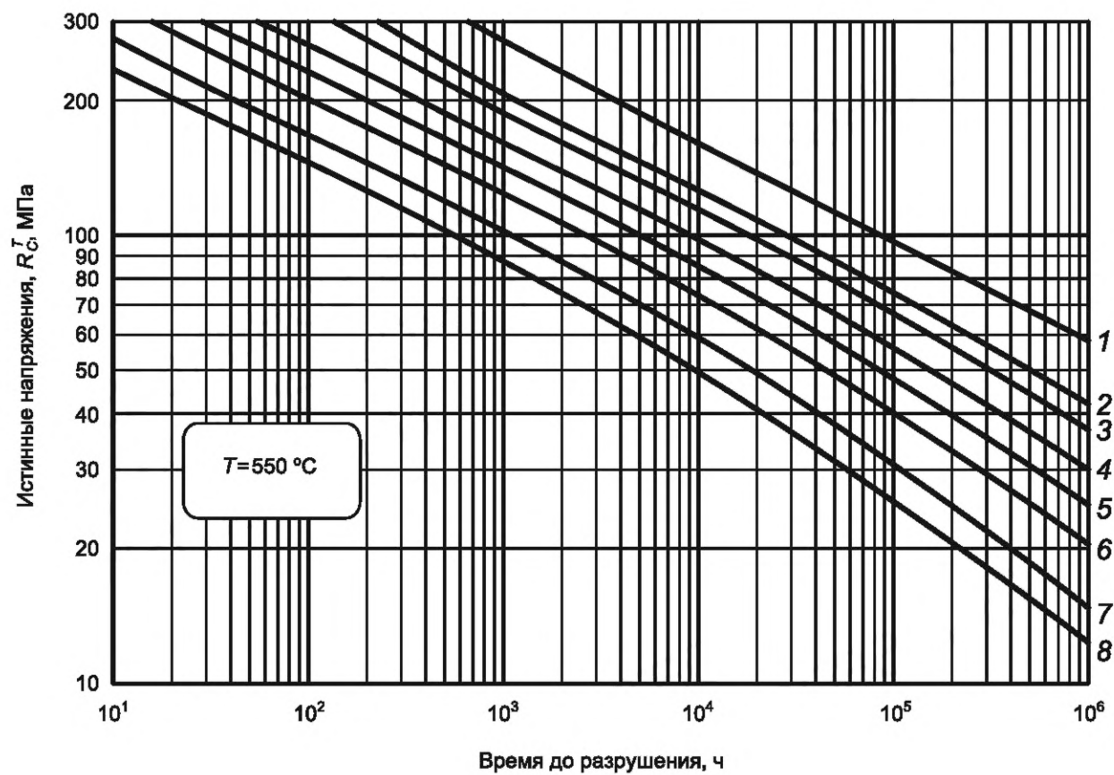
Рисунок В.3 — Кривые минимальных значений истинных напряжений R_c^T сталей марок 09X18H9, 10X18H9, 12X18H9 при различных температурах T и скоростях повреждающей дозы \Phi
