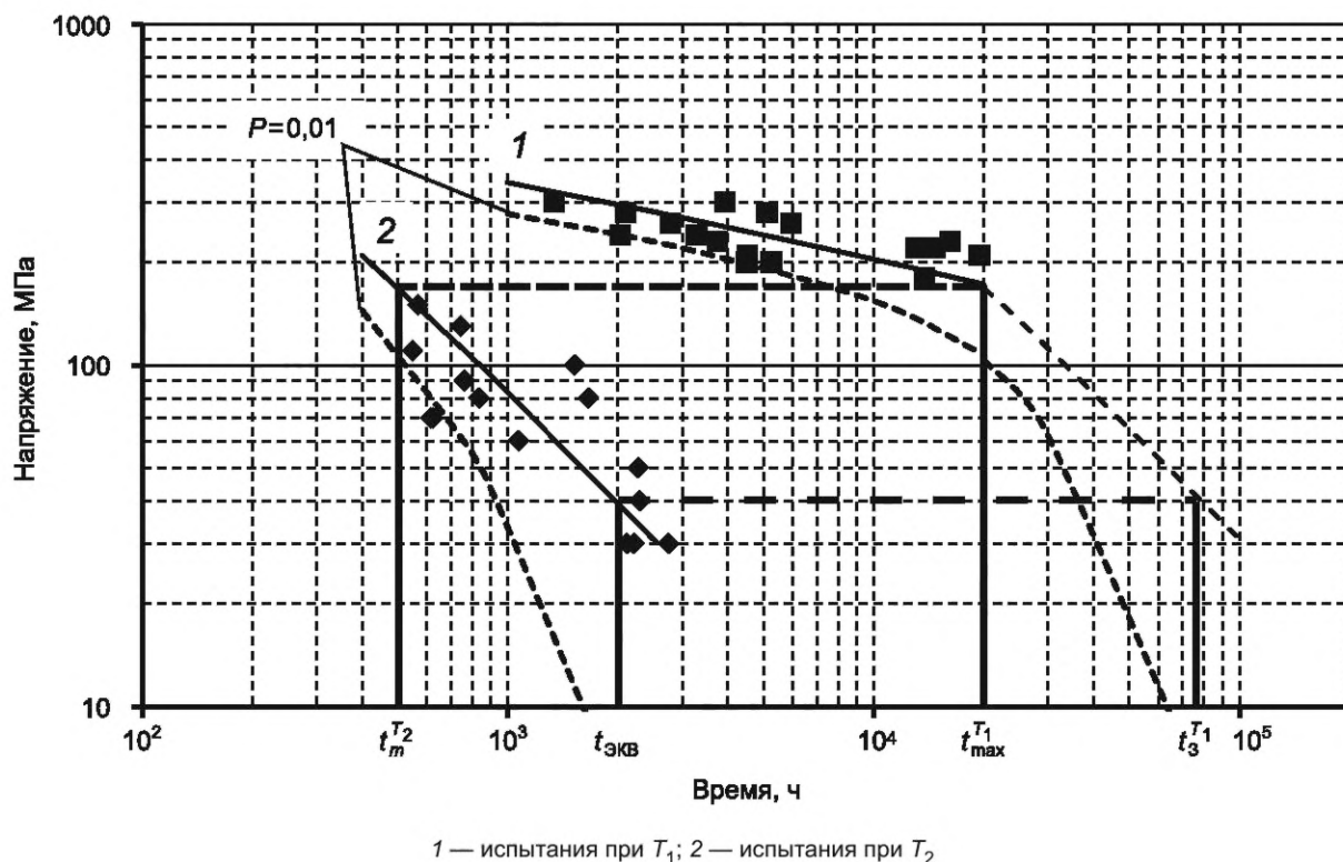
Рисунок 1 — Кривые длительной прочности
