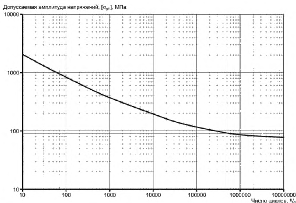
Рисунок А.1 — Расчетная кривая усталости материалов из углеродистых и легированных сталей ( R_{\sigma 0.2}^T / R_m^T \leq 0,7 , R_m^T \geq 450 МПа, Z^T \geq 32\% и E^T \geq 175 ГПа) в интервале температур от 20 °С до 350 °С
