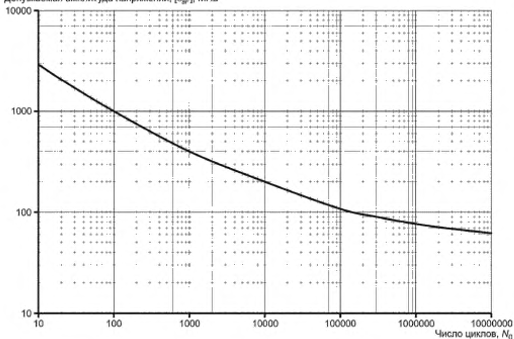
Рисунок А.2 — Расчетная кривая усталости материалов из сталей аустенитного класса ( R_{\text{p0.2}}^T/R_m^T \leq 0.7 , R_m^T \geq 360 МПа, Z^T \geq 45\% и E^T \geq 167 ГПа) в интервале температур от 20 °С до 450 °С
