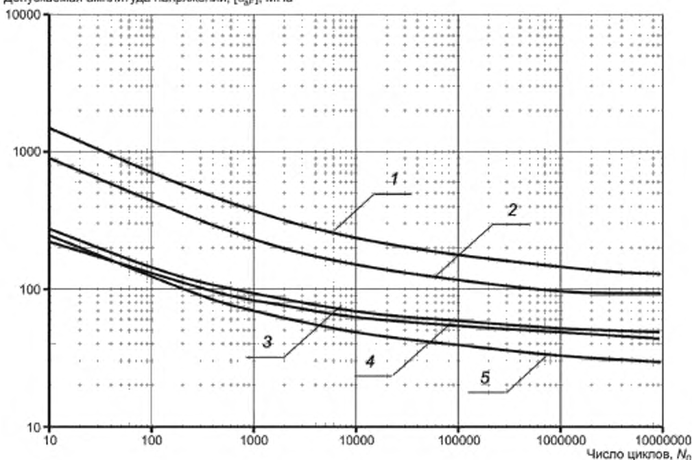
Рисунок А.7 — Расчетные кривые усталости материалов из железоникелевых дисперсионно-твердеющих сплавов (ХН35ВТ) при длительности нагружения 2 \cdot 10^5 ч
