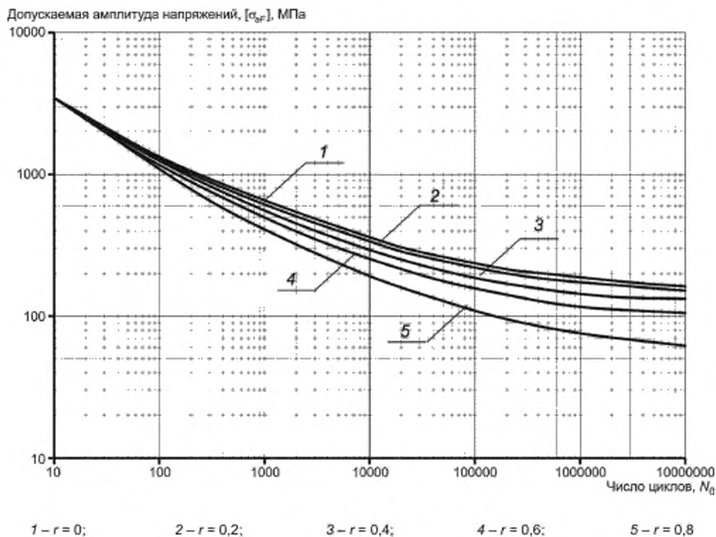
Рисунок А.4 — Расчетные кривые усталости для резьбовых участков шпилек и болтов из сталей перлитного класса с R_{\text{тл}} \geq 760 МПа до температуры T = 350 °С при различных значениях коэффициента асимметрии r
