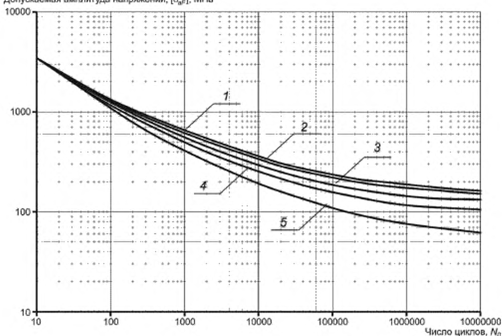
Рисунок А.5 — Расчетные кривые усталости материалов из легированных сталей при длительности нагружения 2 \cdot 10^5 ч
