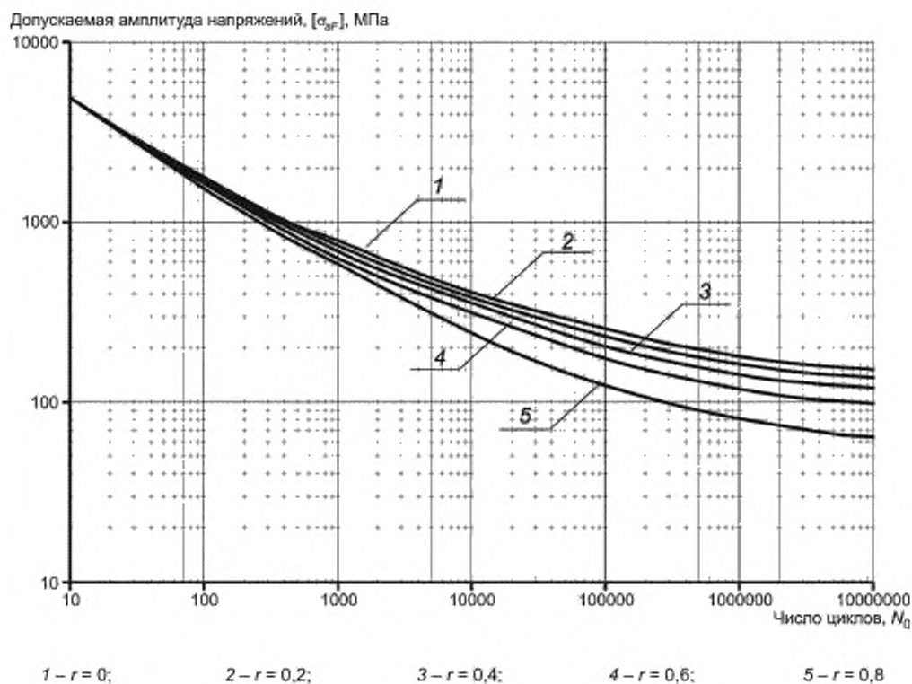
Рисунок А.3 — Расчетные кривые усталости для резьбовых участков шпилек и болтов из сталей перлитного класса с 660 \leq R_m^T < 760 МПа до температуры T = 350 °C при различных значениях коэффициента асимметрии r
