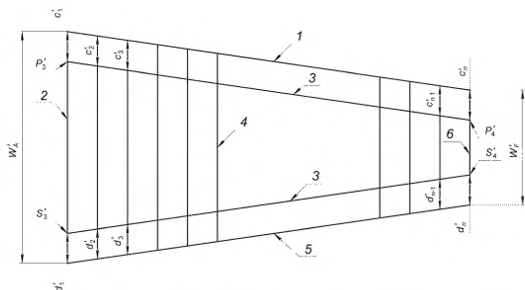
1 — переборка правого борта; 2 — кормовая поперечная переборка; 3 — продольные горизонтальные опоры; 4 — поперечное сечение танка; 5 — переборка левого борта; 6 — носовая поперечная переборка; W_A — ширина по кормовой поперечной переборке; W_F — ширина по носовой поперечной переборке; P'_i, S'_i — точки измерения на поперечных переборках; c'_1 \dots c'_n и d'_1 \dots d'_n — расстояния между продольными опорами и соответствующими бортовыми переборками
