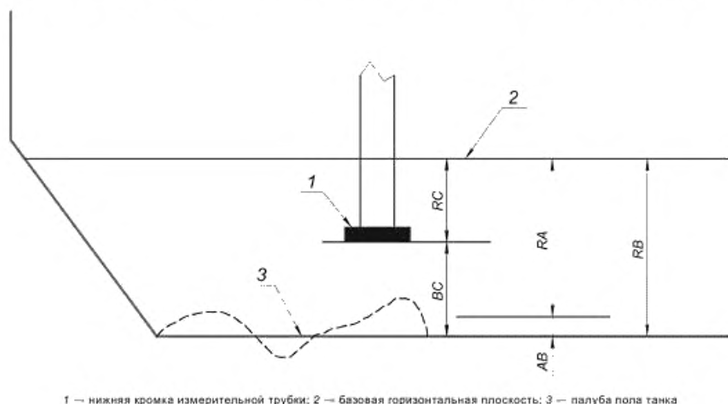
Рисунок 6 — Схема донной части танка
