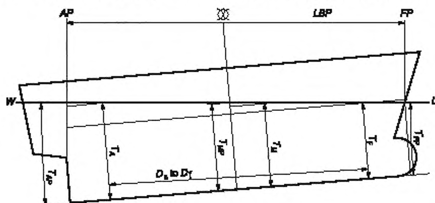
Рисунок 1 — Отстояние марок углублений от перпендикуляров
