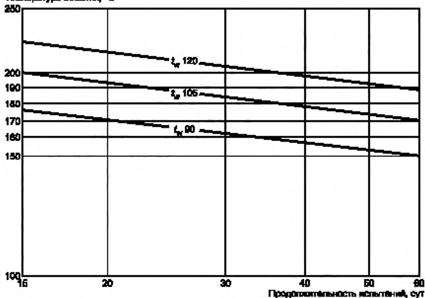
Рисунок U.1 — Зависимость между температурой обмотки и продолжительностью длительных испытаний
