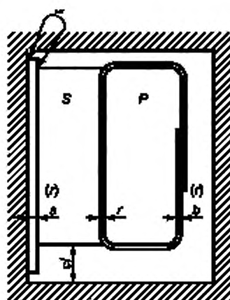
Первичная или вторичная обмотка, обернутая изоляционным материалом Класс I (II) М.2.1 c)
