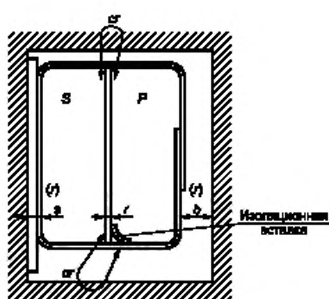
Первичная и вторичная обмотки, обернутые изоляционным материалом (нет путей утечки) Класс I (II) М.2.1 d)
