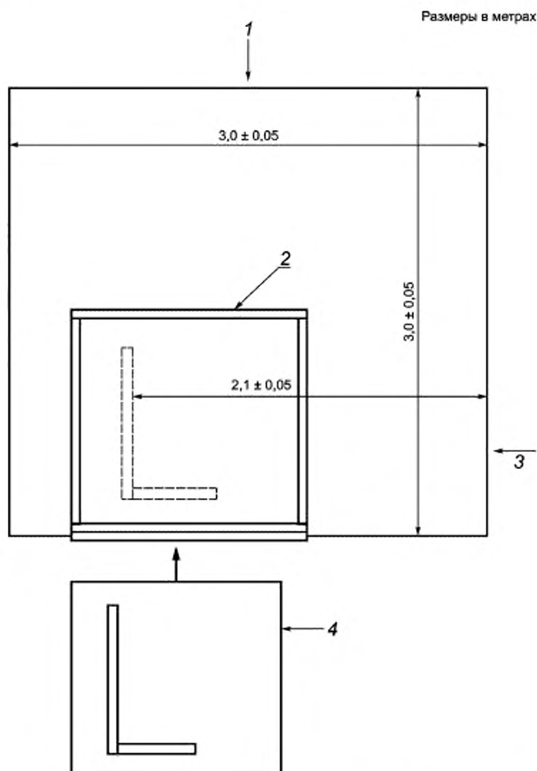
1 — смотровое окно; 2 — неподвижная рама; 3 — смотровое окно (с ориентированным влево образцом), 4 — тележка для образцов (с ориентированным влево образцом)
