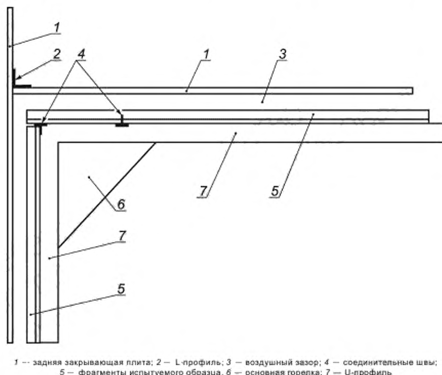
Рисунок 2 — Пример монтажа образца
