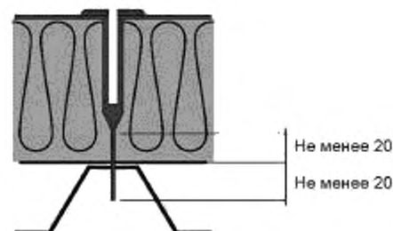
Рисунок 11 — Установка телескопического крепежа в несущее основание из профилированного настила
