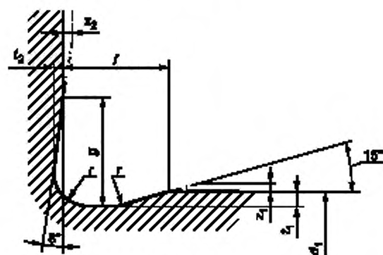
d_1 — диаметр заготовки; f — ширина поднутрения; r — радиус поднутрения; t_1, t_2 — глубина поднутрения; z_1, z_2 — припуск на обработку
