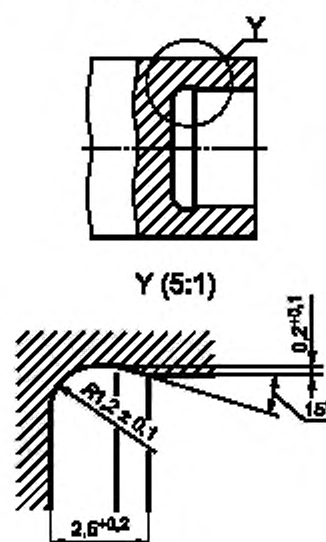
Рисунок 8 — Упрощенные данные о поднутрении E 1,2 × 0,2
