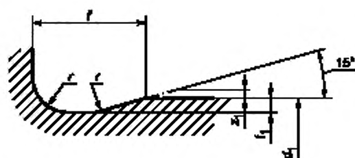
d_1 — диаметр заготовки; f — ширина поднутрения; r — радиус поднутрения; t_1 — глубина поднутрения; z_1 — припуск на обработку
