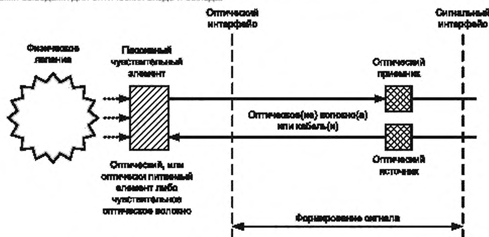
Рисунок А.1 — Конфигурация ВОД с пассивным чувствительным элементом и отдельными волоконными выводами для оптических входа и выхода
