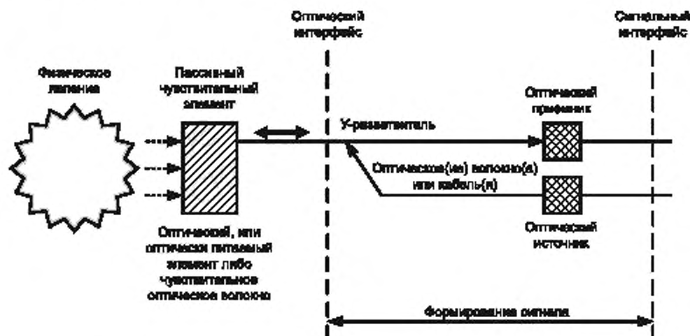
Рисунок А.3 — Конфигурация ВОД с пассивным чувствительным элементом и одним волоконным выводом для оптических входа и выхода
